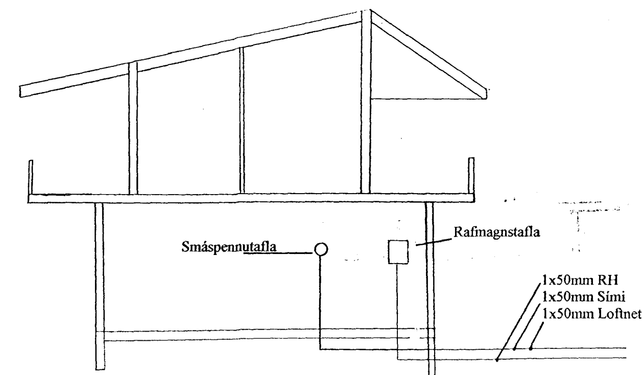
1:100 Inntakspípur 70 sm í jörð 3x50mm. Að lóðarmörkum.
