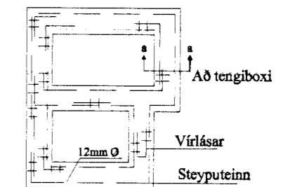
Grunnmynd sökkulvegga
