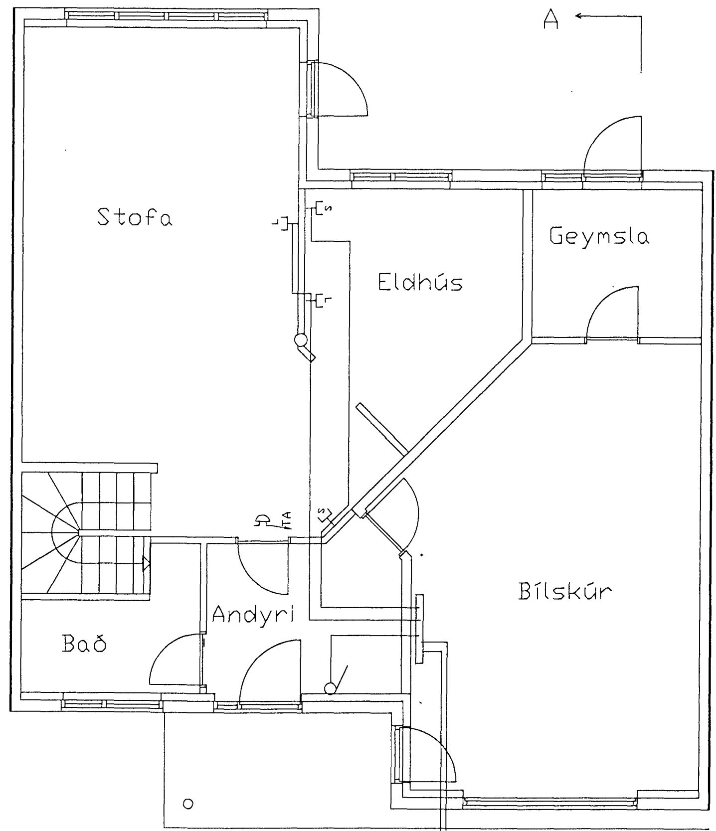
Grunnmynd 1.Hæð
