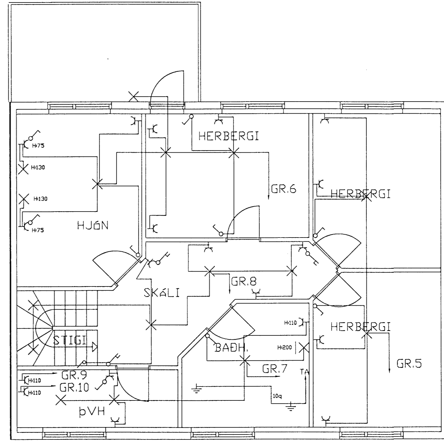
○ Grunnmynd 2.Hæð
