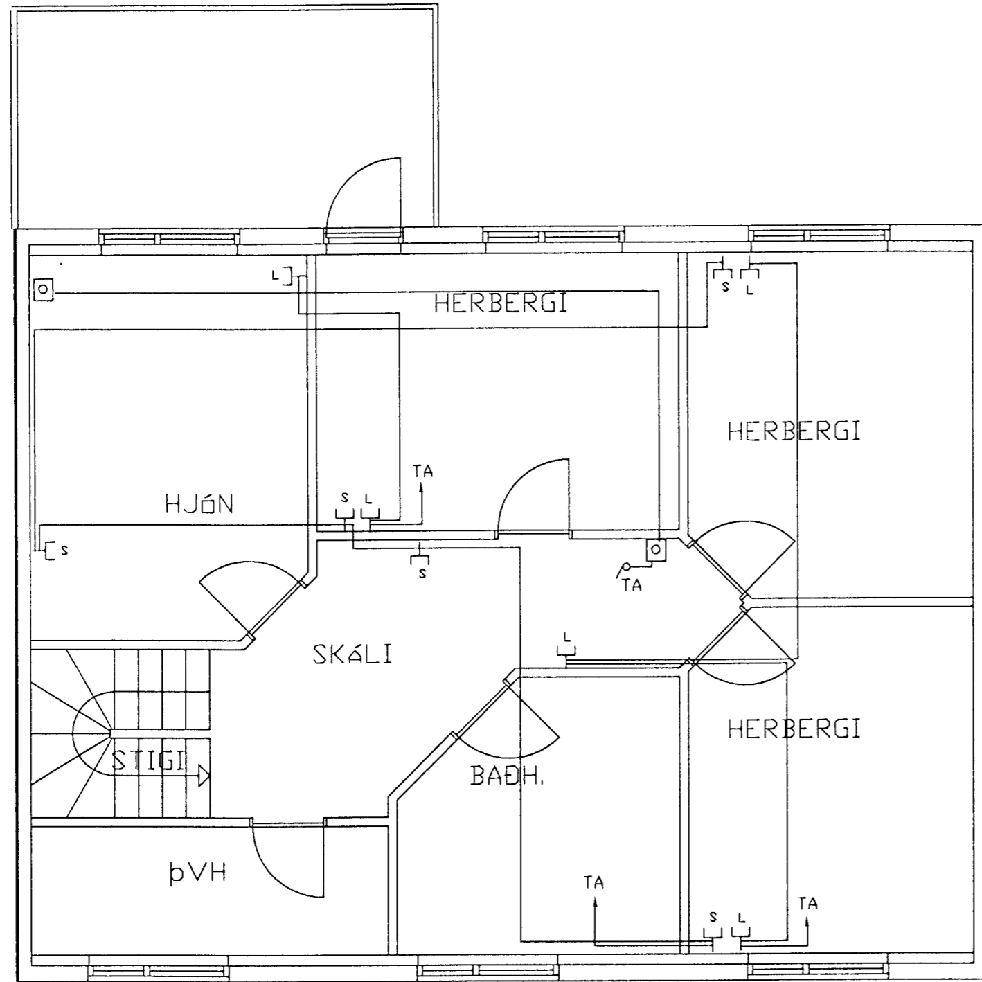
○ Grunnmynd 2.Hæð
