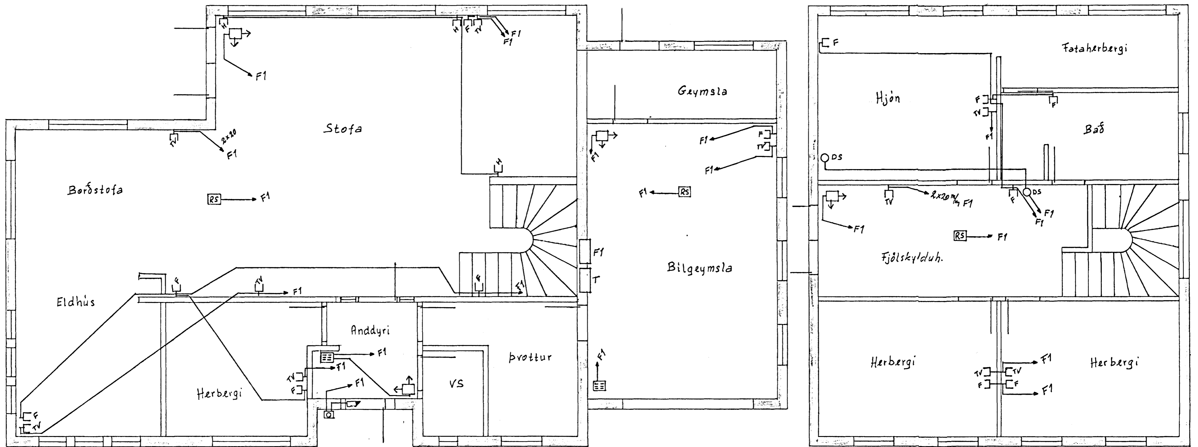
II - Hæð
