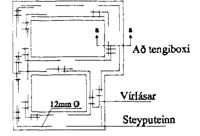
Grunnmynd sökkulveggja
