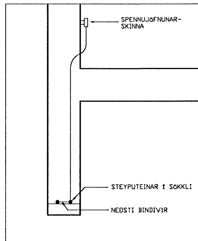
TENGING SÖKKULSKAUTS DÆMIGERÐUR FRÁGANGUR
