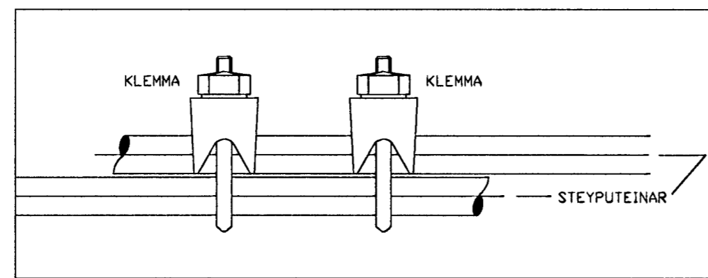
SAMTENGING TEINA DÆMIGERÐUR FRÁGRANGUR
