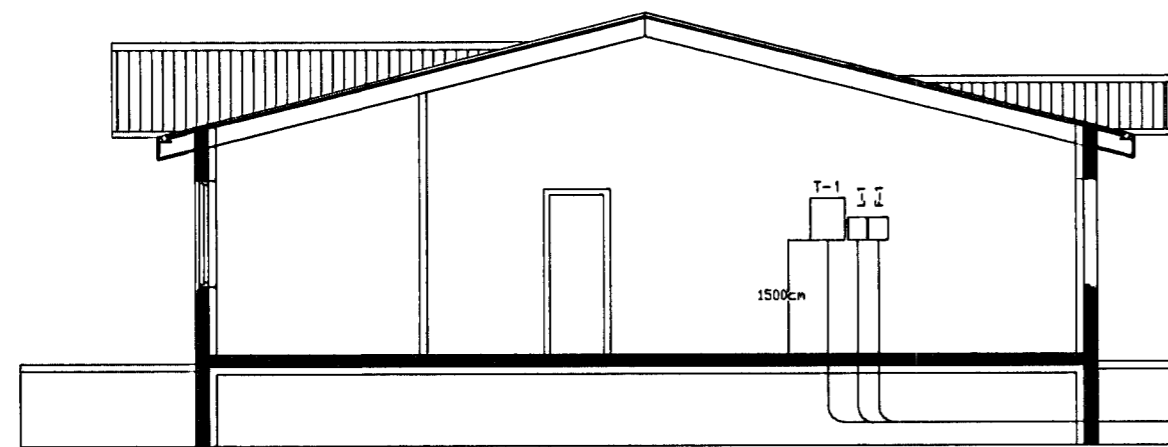
Skurður C-C, Mkv. 1 : 100
