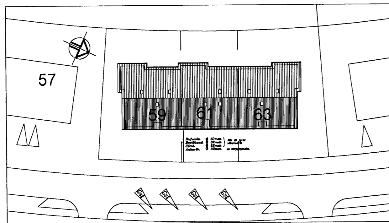
Afstöðumynd Mkv 1:500
