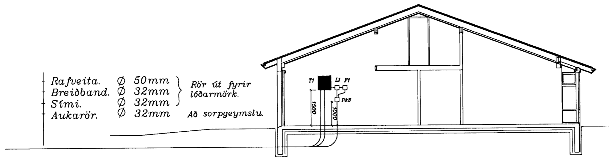
Snið Mkv 1 : 100
