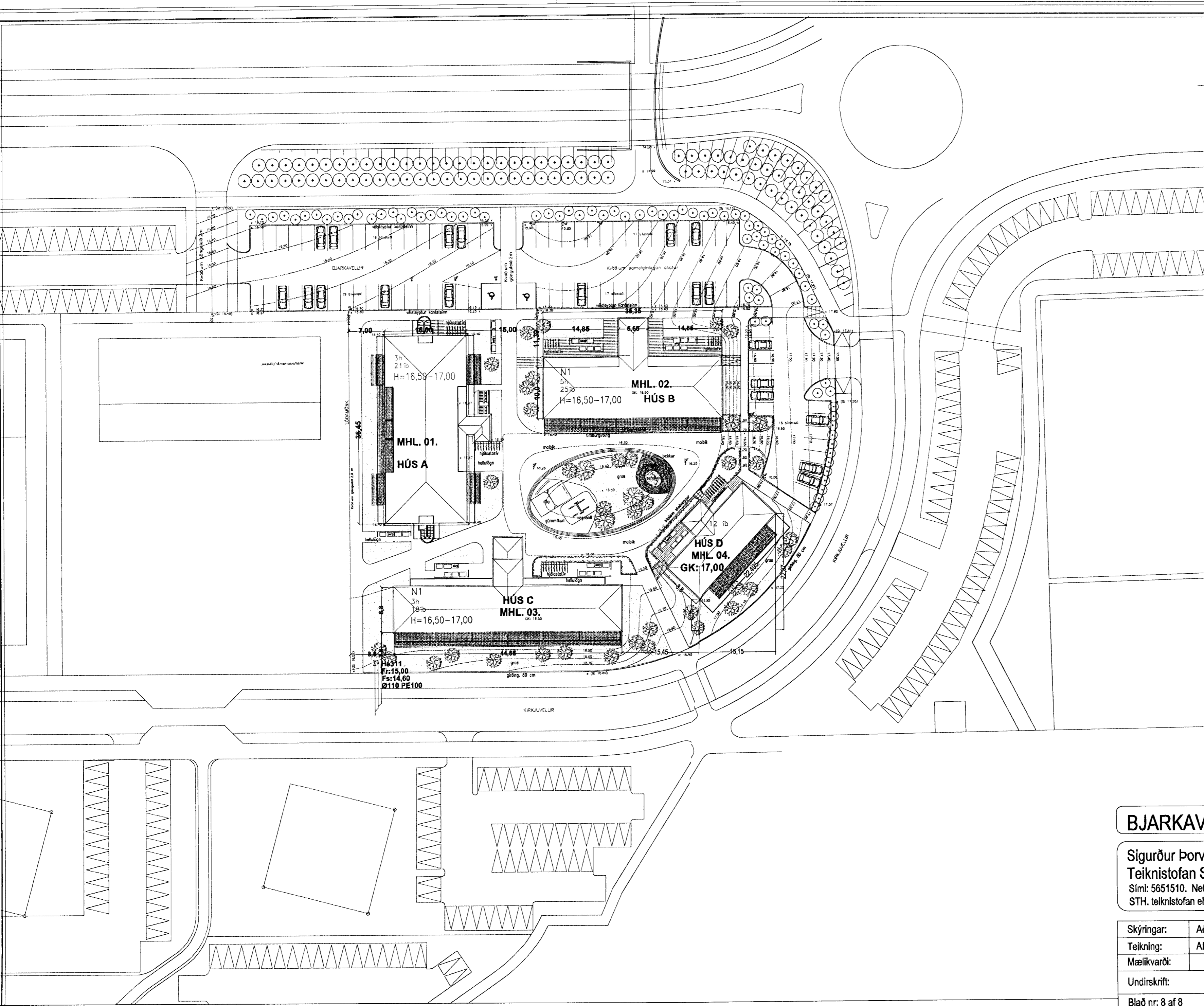
AFSTÖÐUMYND. MKV. 1:500.
