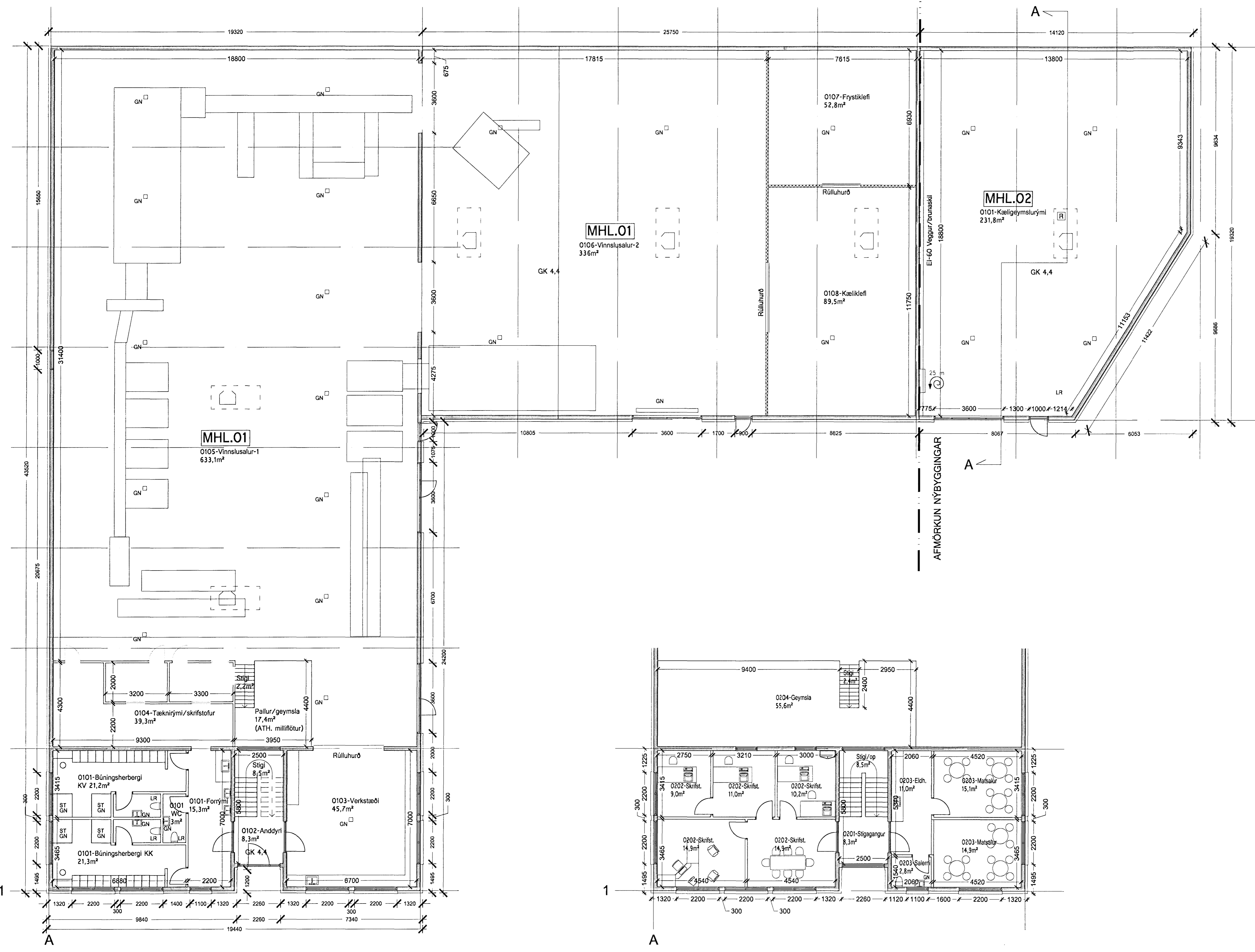
GRUNNMYND 1. HÆÐ MKV 1:100
