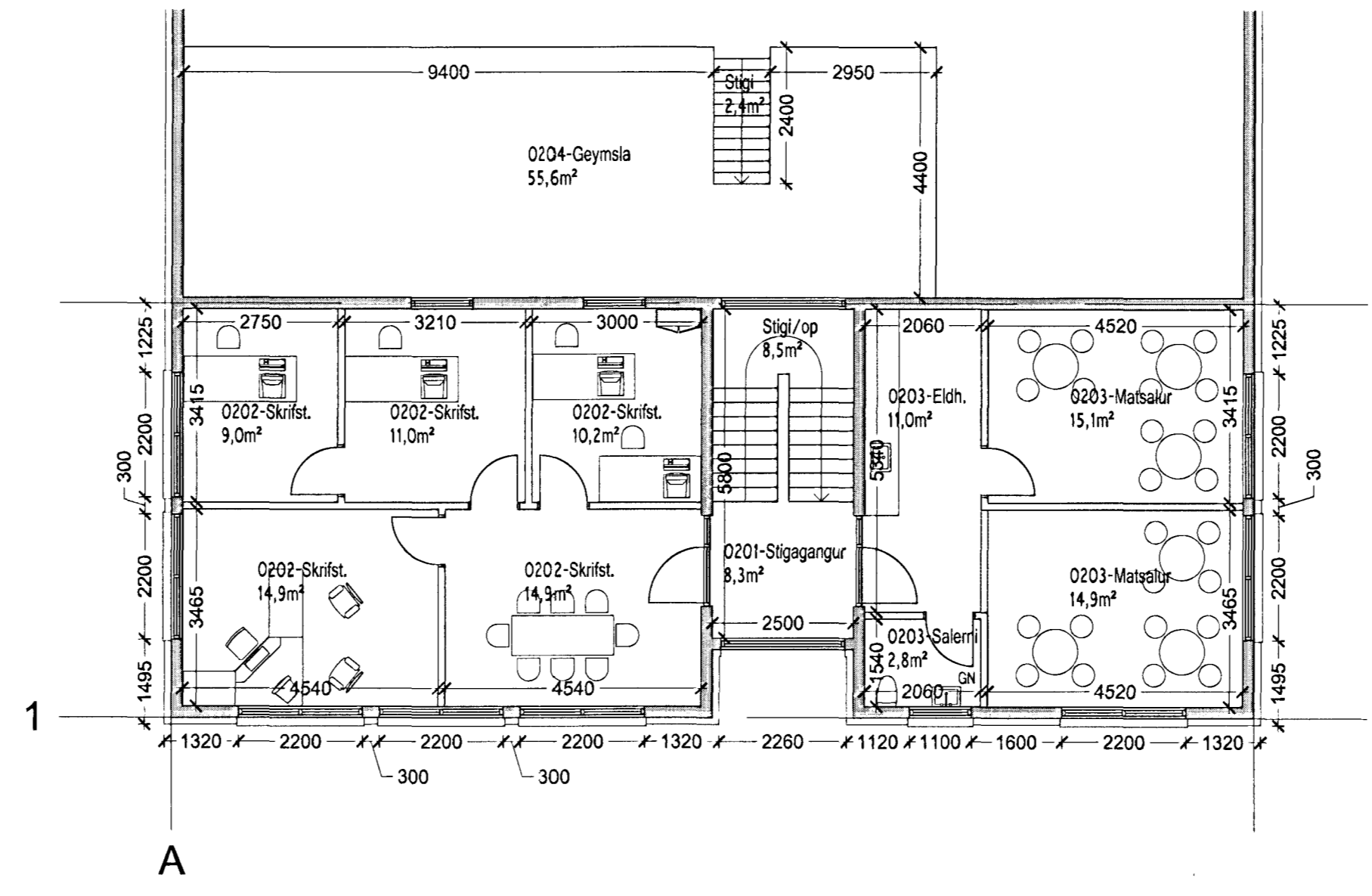
GRUNNMYND 2. HÆÐ MKV 1:100
