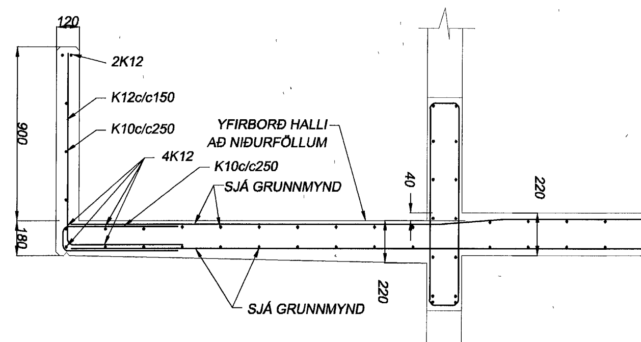
SNID Í SVALIR, 1:20
