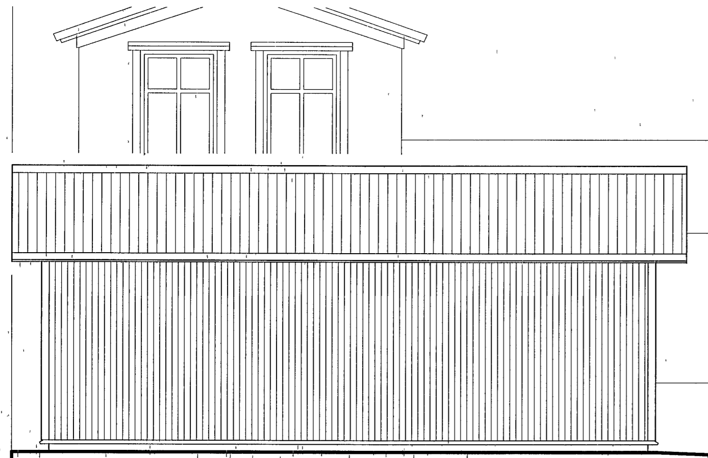
Ásýnd - Norður mkv. 1:50
