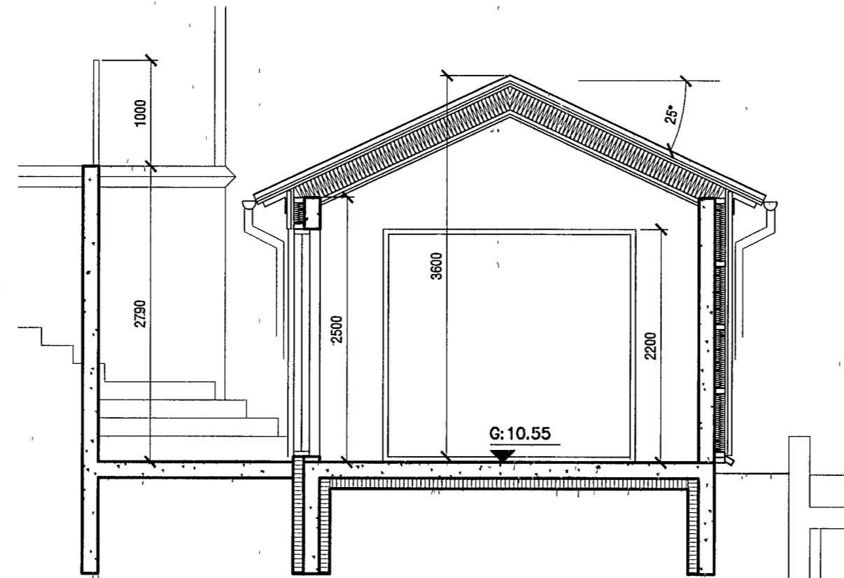
Sneiðing A-A mkv. 1:50
