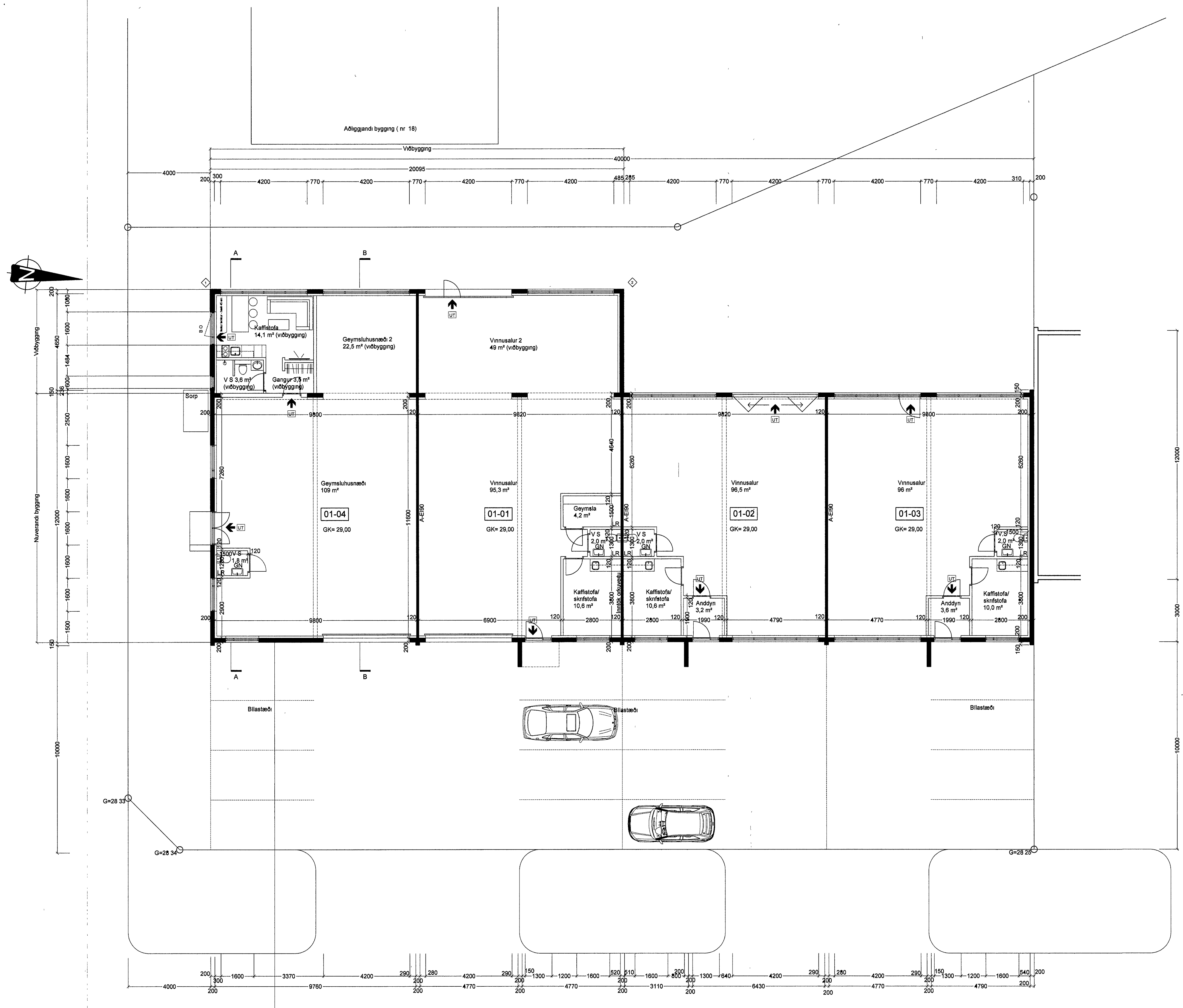
Grunnmynd 1. hæðar 1:100
