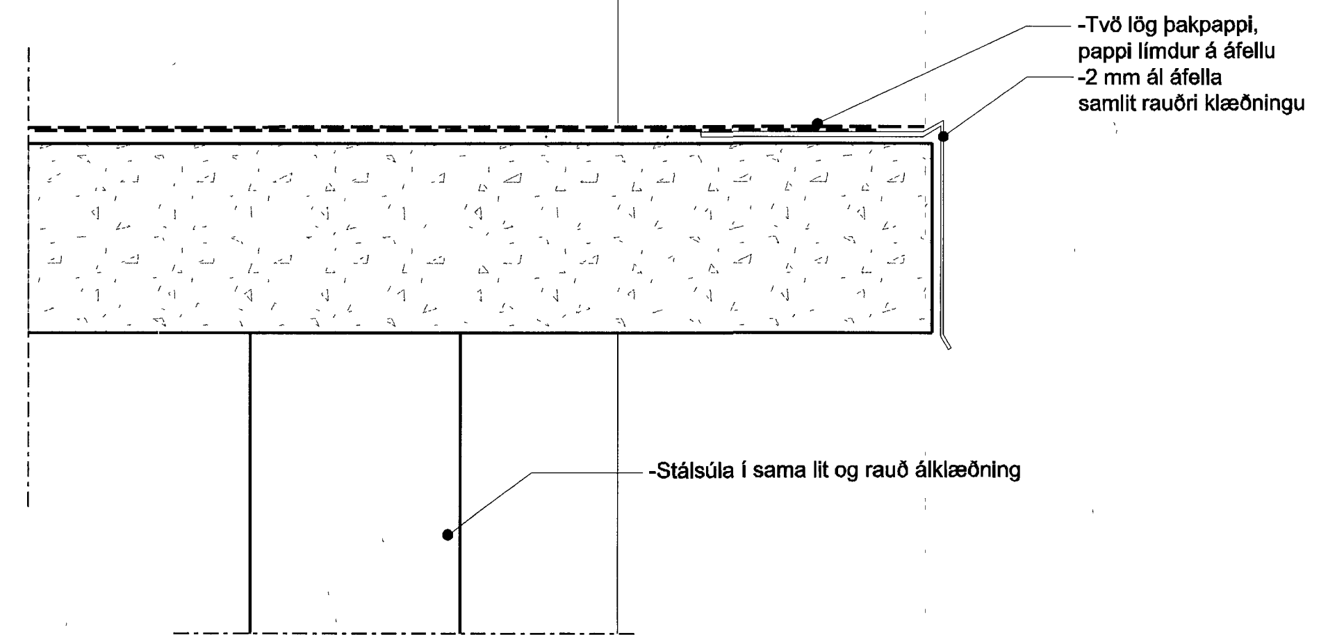
6 - DEILI 1:5 Frágangur á skyggni við aðallíngang
