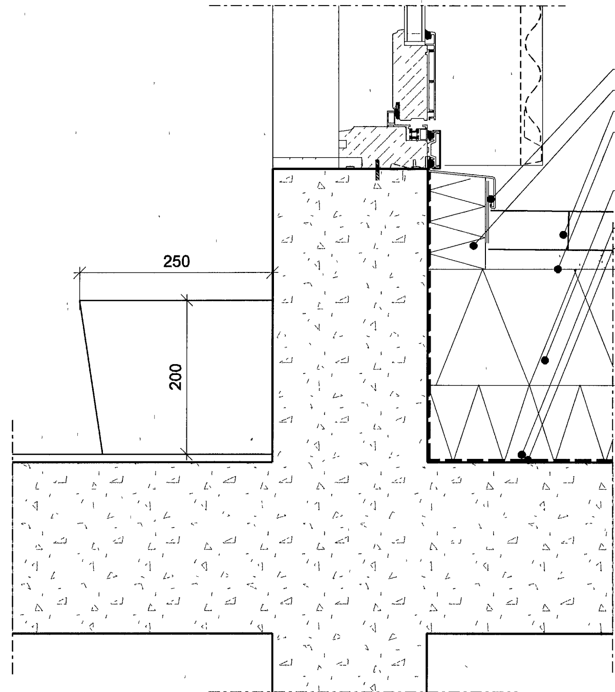
1 - DEILI 1:5 Svaladyr og svalfrágangur á 5. hæð
