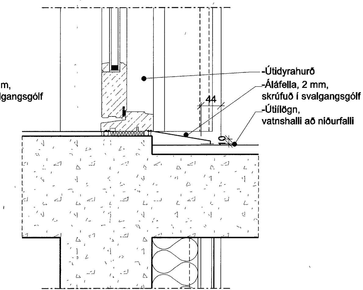
3 - DEILI 1:5 Botnstykki útidyráhrúa við svalgang
