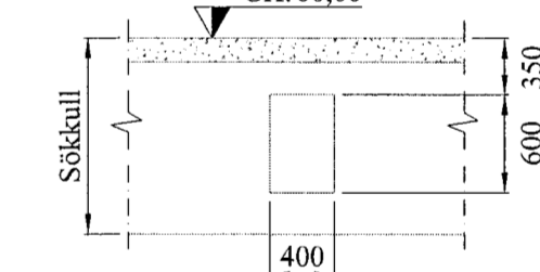
Skýringamynd af inntaksgati GK:00,00
