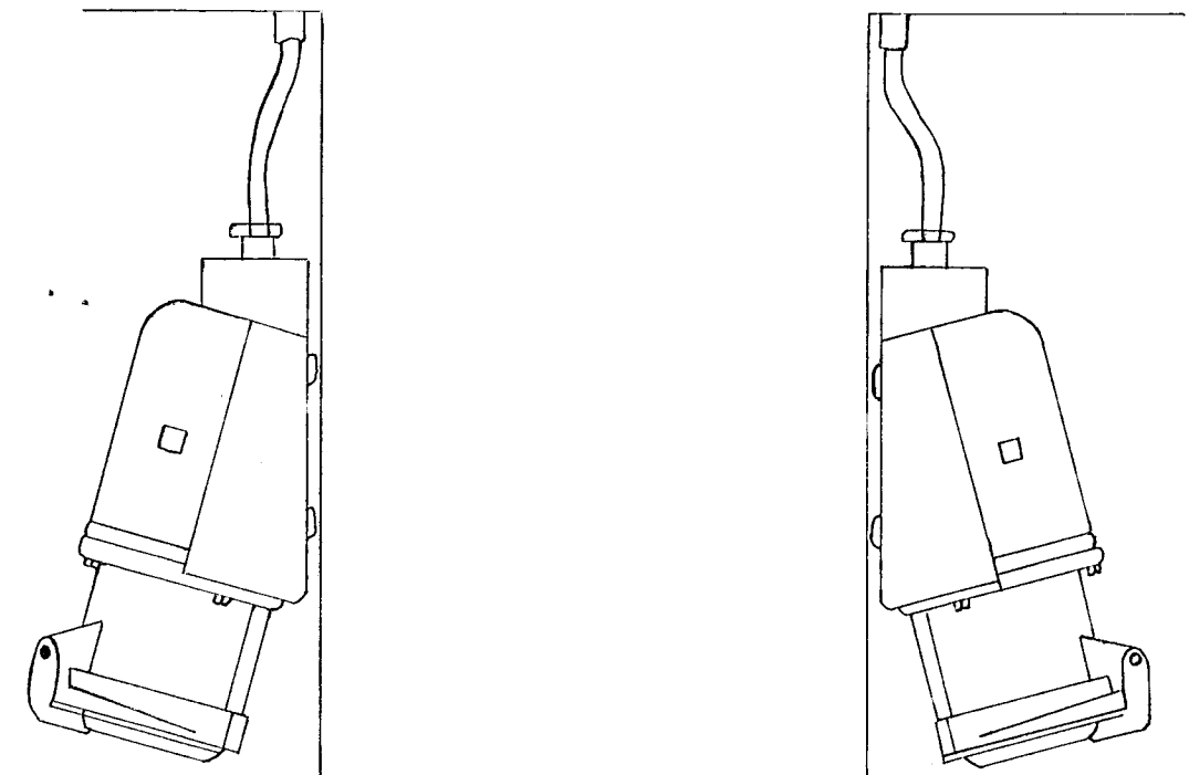
SKURÐUR A-A.
