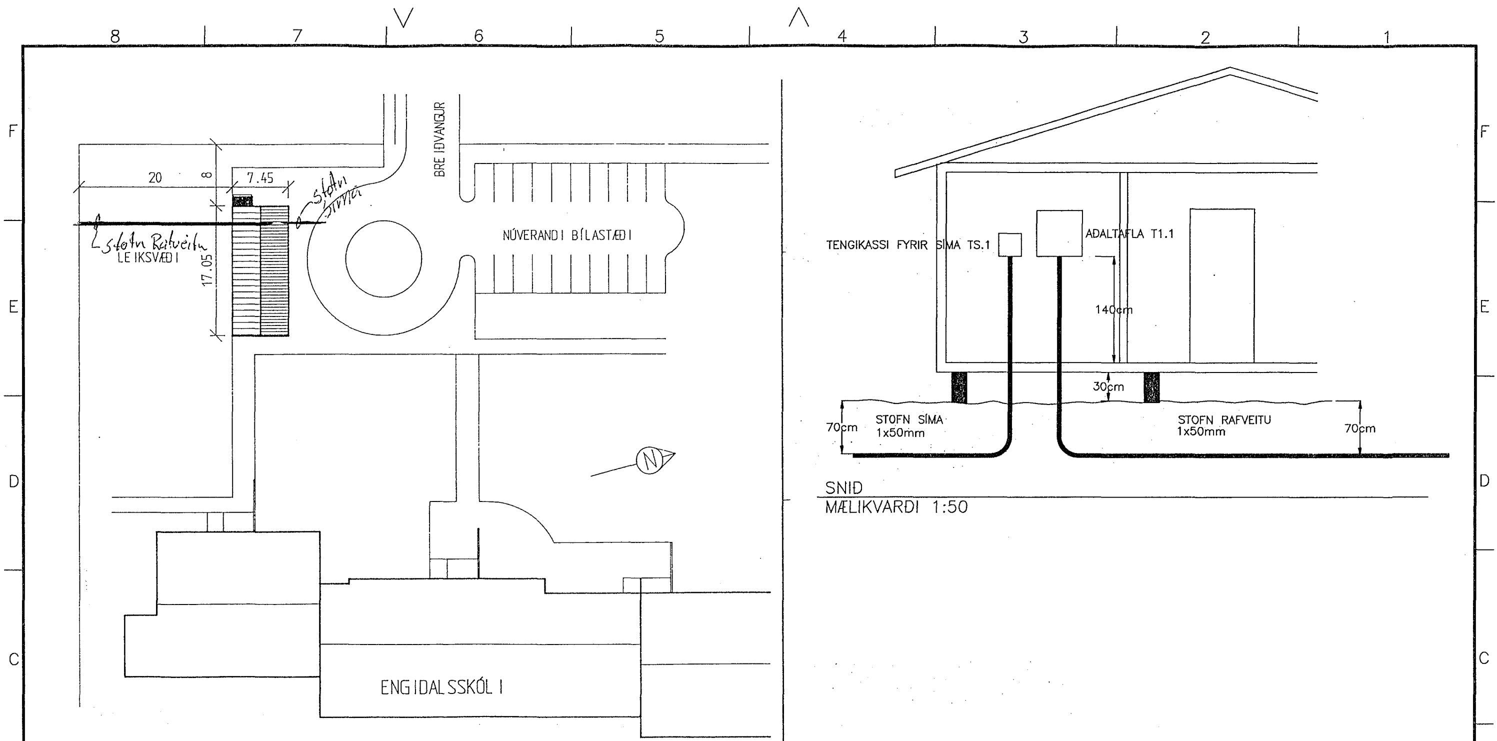
AFSTÖDUMYND MÆLIKVARDI 1:500
