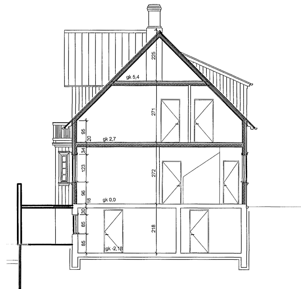
3 SNID B-B 1:100
