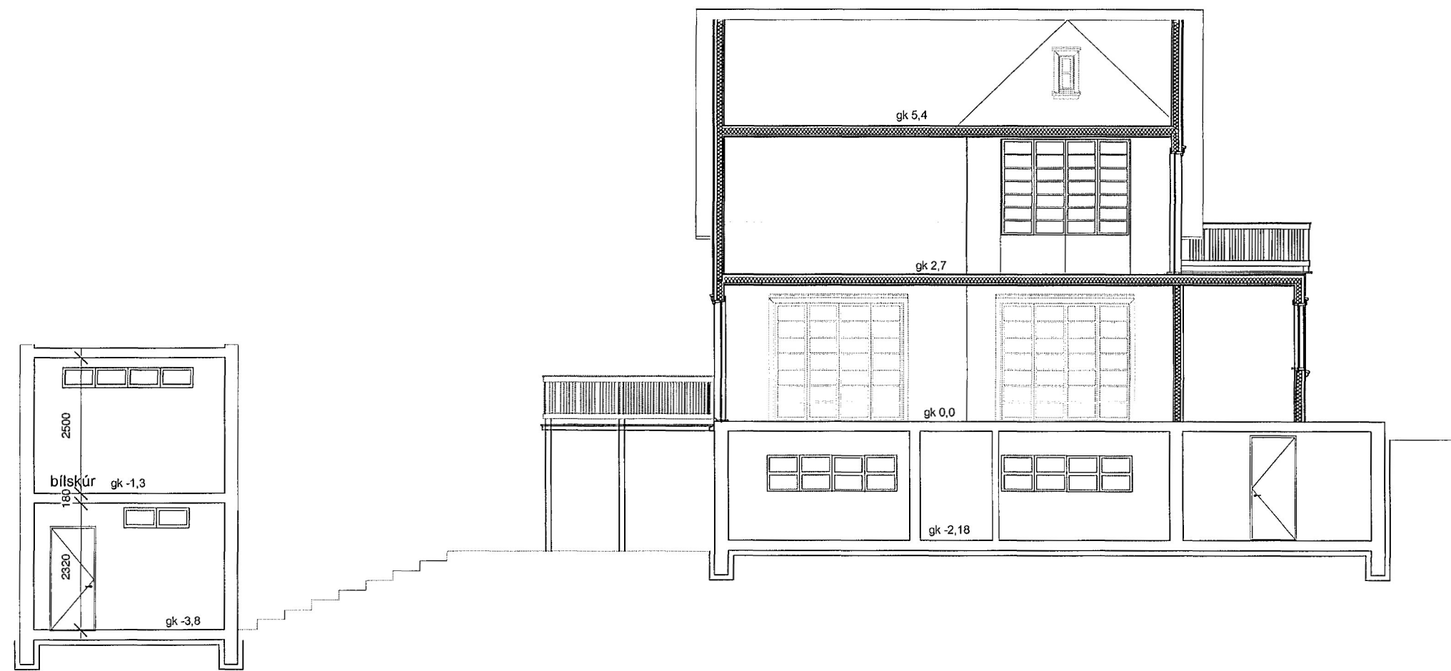
3 SNID A-A 1:100
