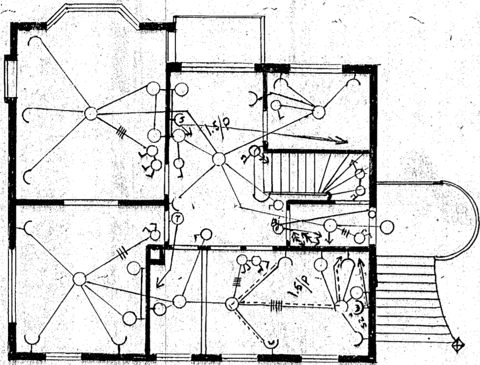
1. HÆÐ.
