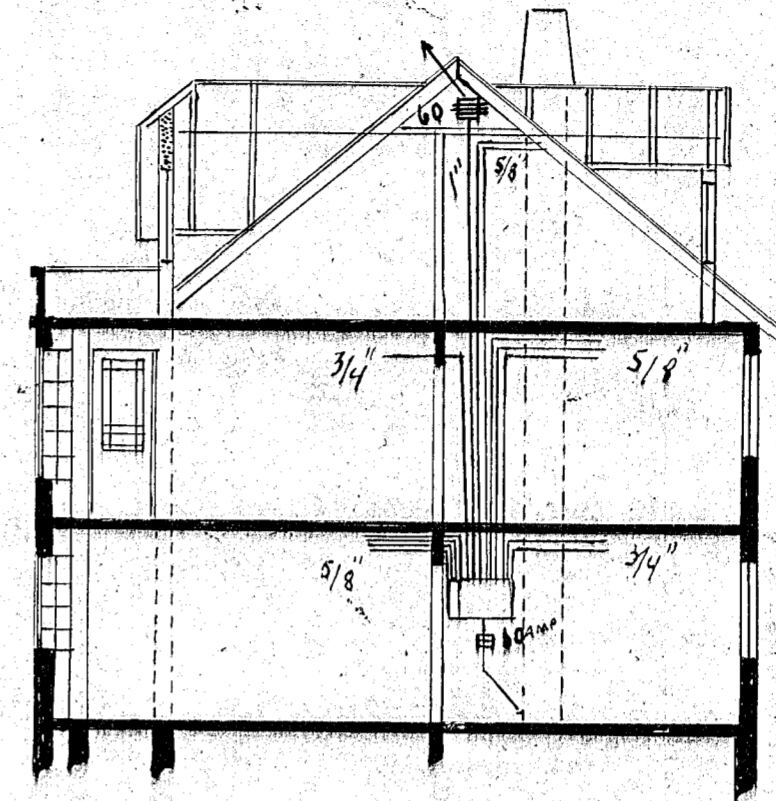
ÞVERSURÐUR.
