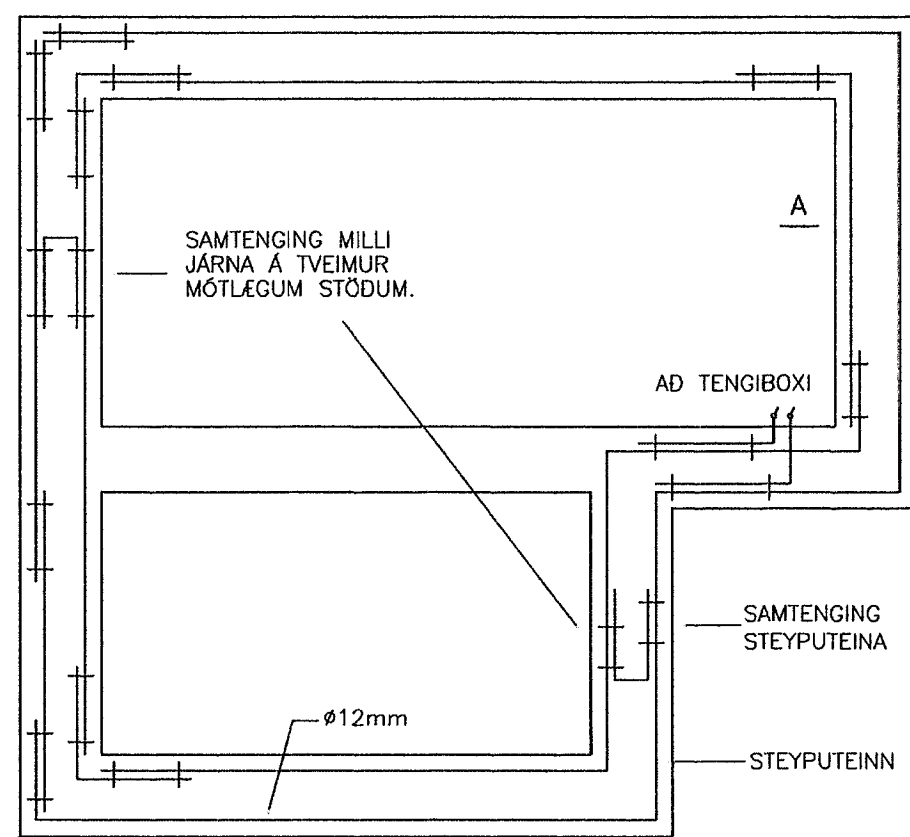
GRUNNMYND SÖKKULVEGGJA
