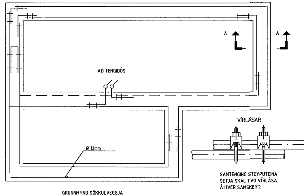
GRUNNMYND SÖKKULVEGGJA DÆMIGERÐ MYND
