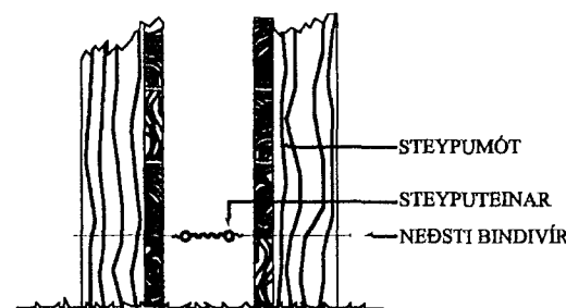
FRÁGANUR Á SAMTENGINUM STEYPUÞEINNA FYRIR SÖKKULJARÐSKAUT
