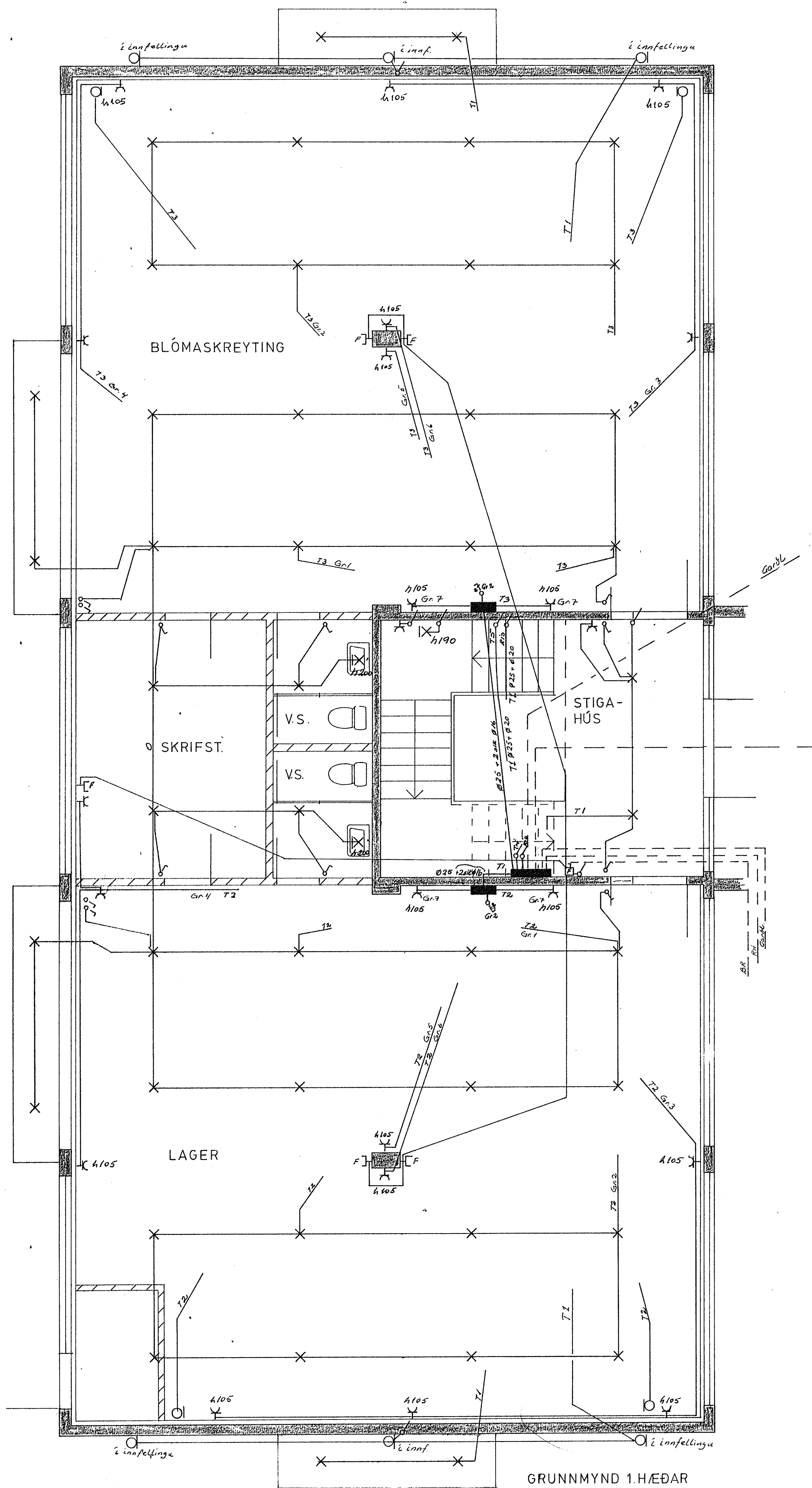
GRUNNMYND 1.HÆÐAR
