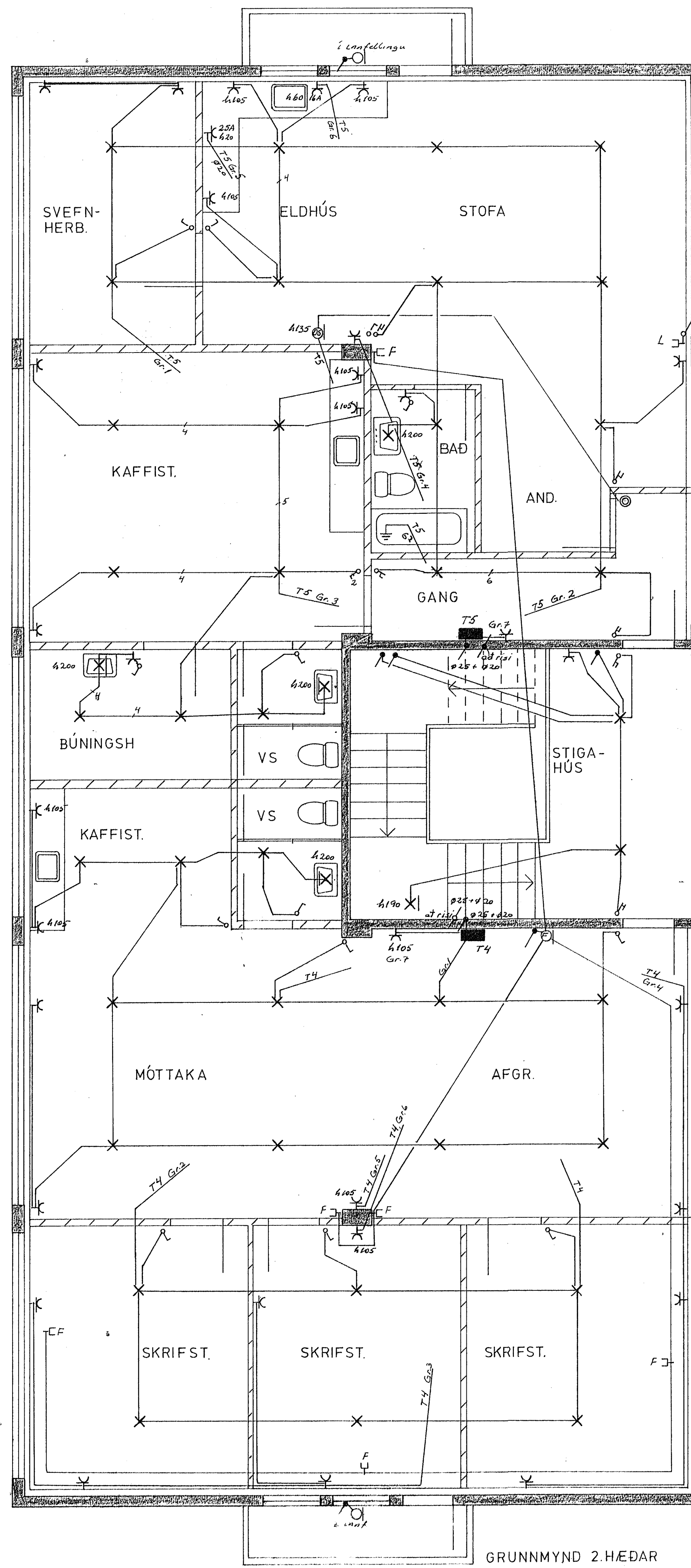
GRUNNMYND 2.HÆÐAR
