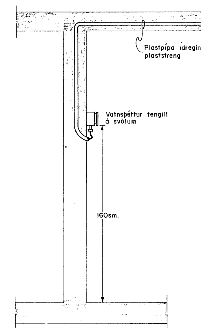
SNID C - C (GILDIR EINNIG F. I. HÆÐ) M. 1:20
