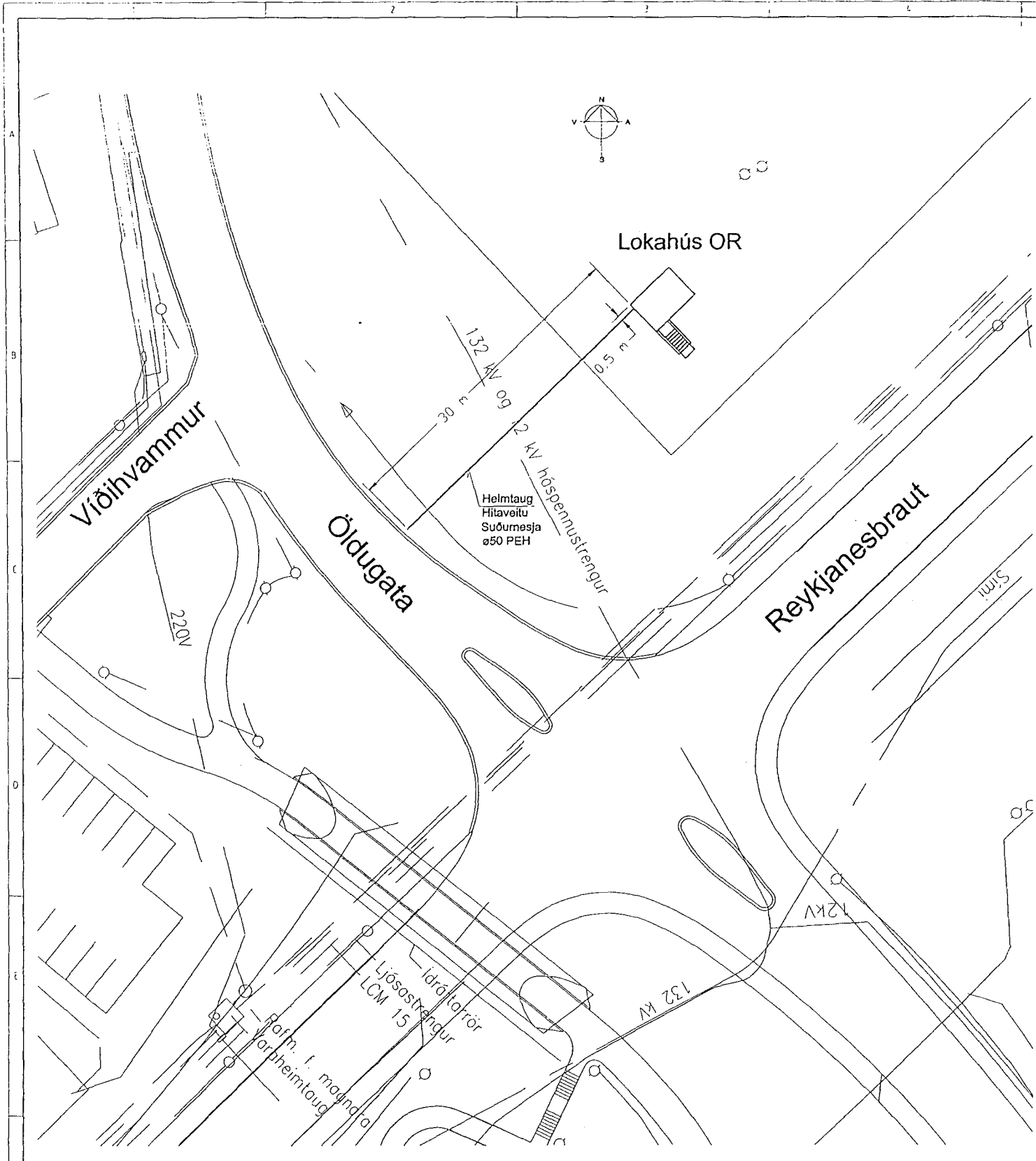
Afstöðumynd Mælikvarði 1:500
