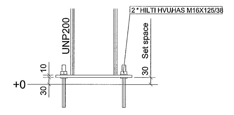
Column foot (D)
