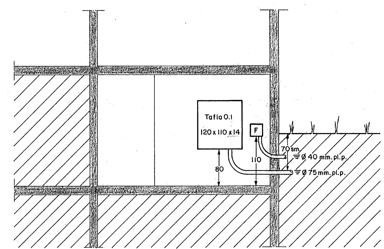
SNID A-A Í INNTAK M. 1:50
