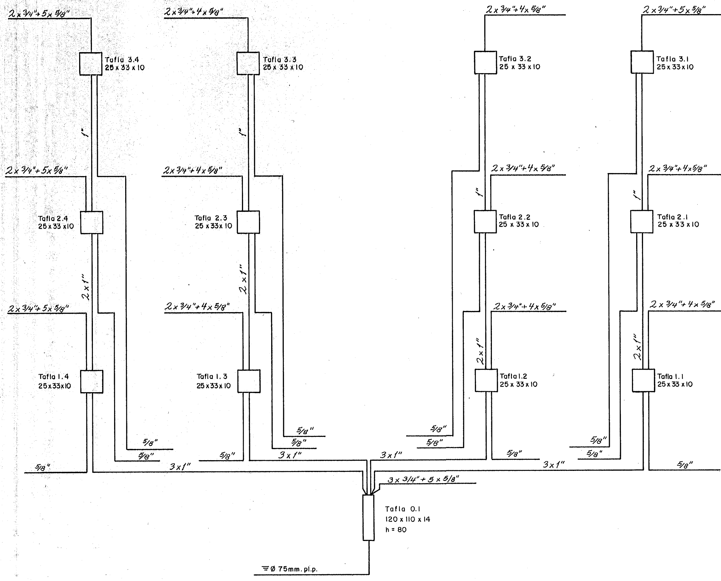
KASSAR OG PÍPUR
