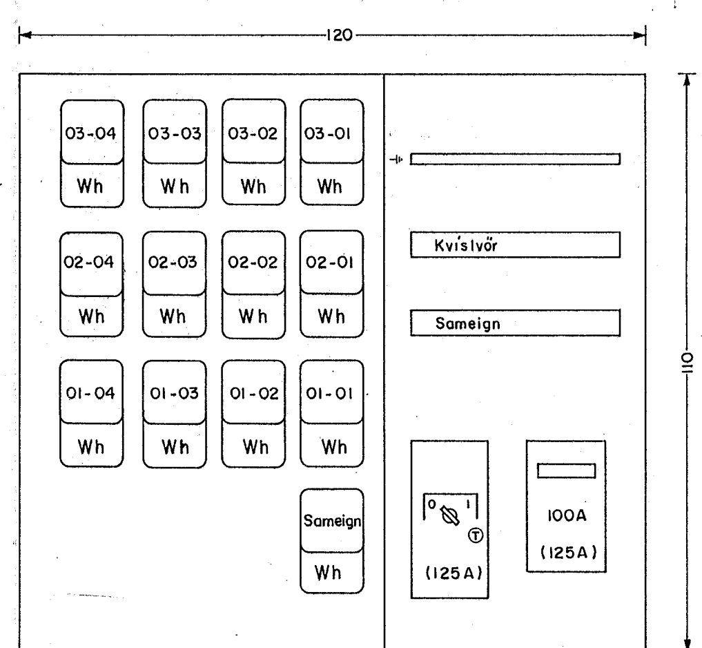
ÚTLIT AF TÖFLU 0.1 M. 1:10
