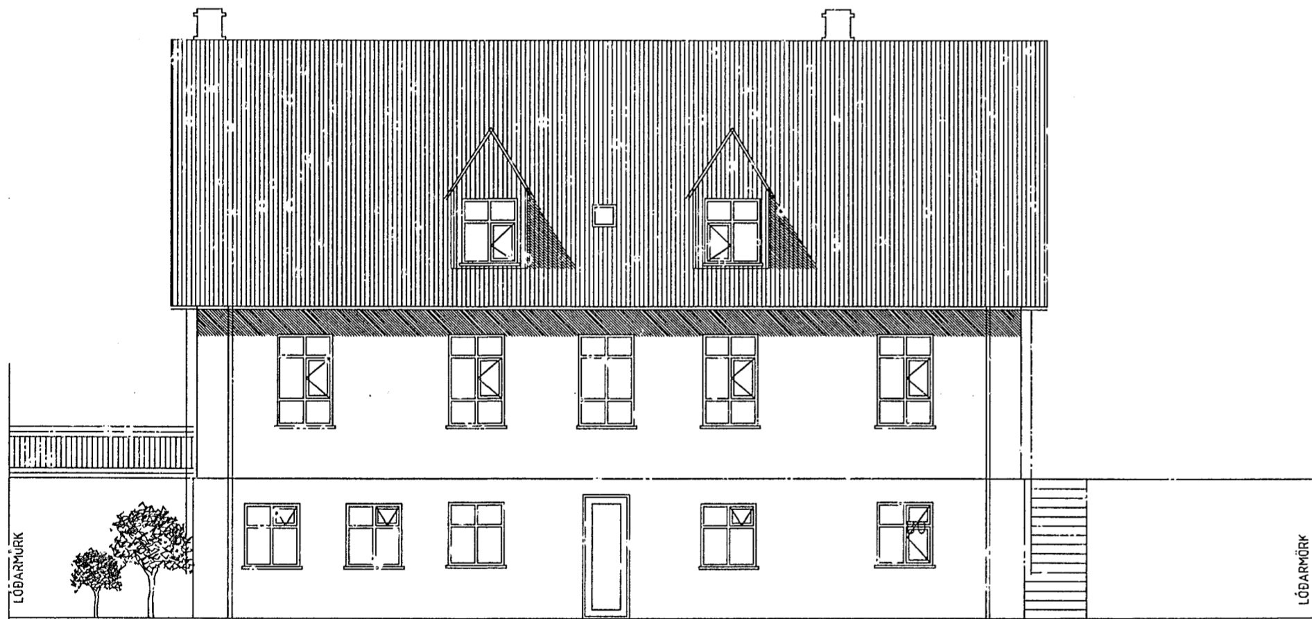
ÚTLIT SUÐVESTUR 1:100
