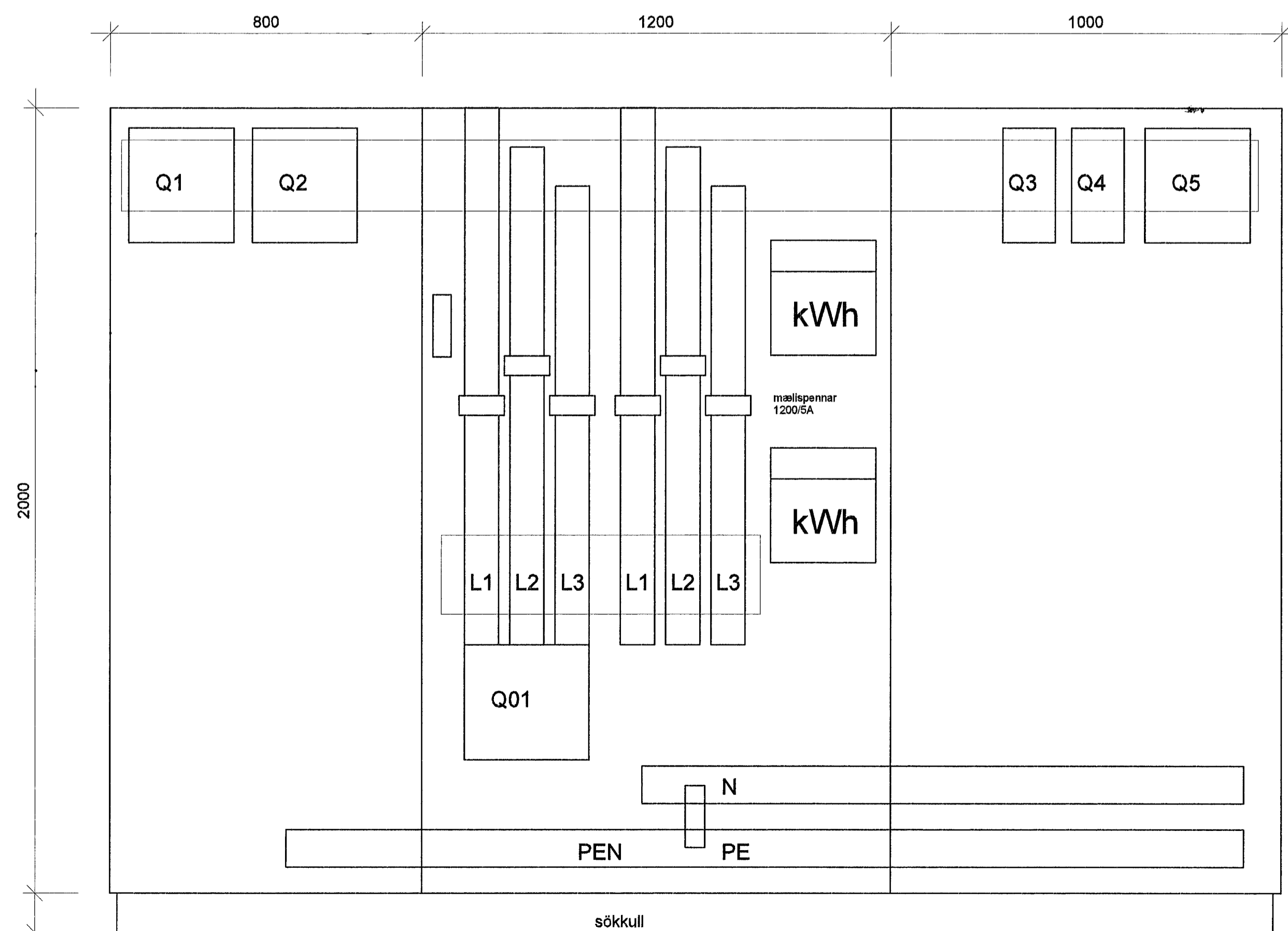
Útlit Aðaltafli mkv 1:10
