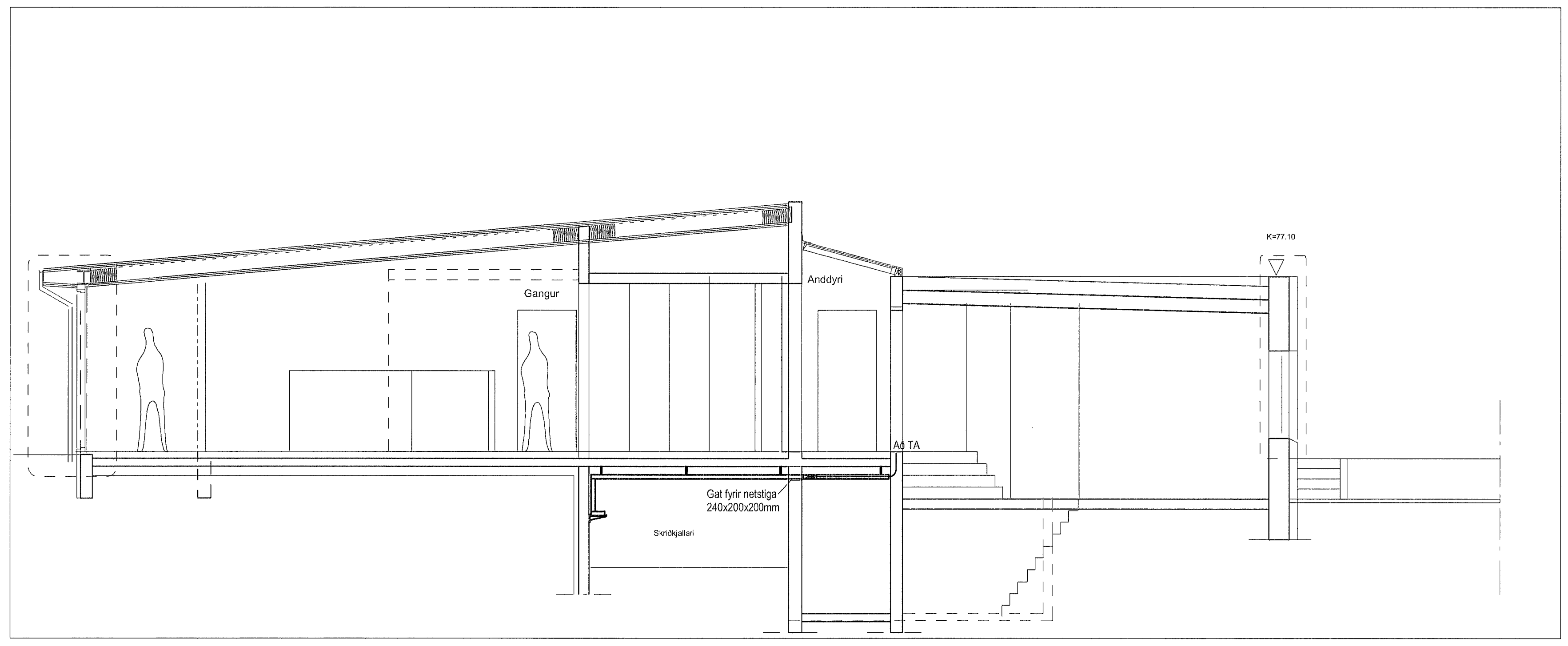
Sniðmynd A-A, mkv. 1:50
