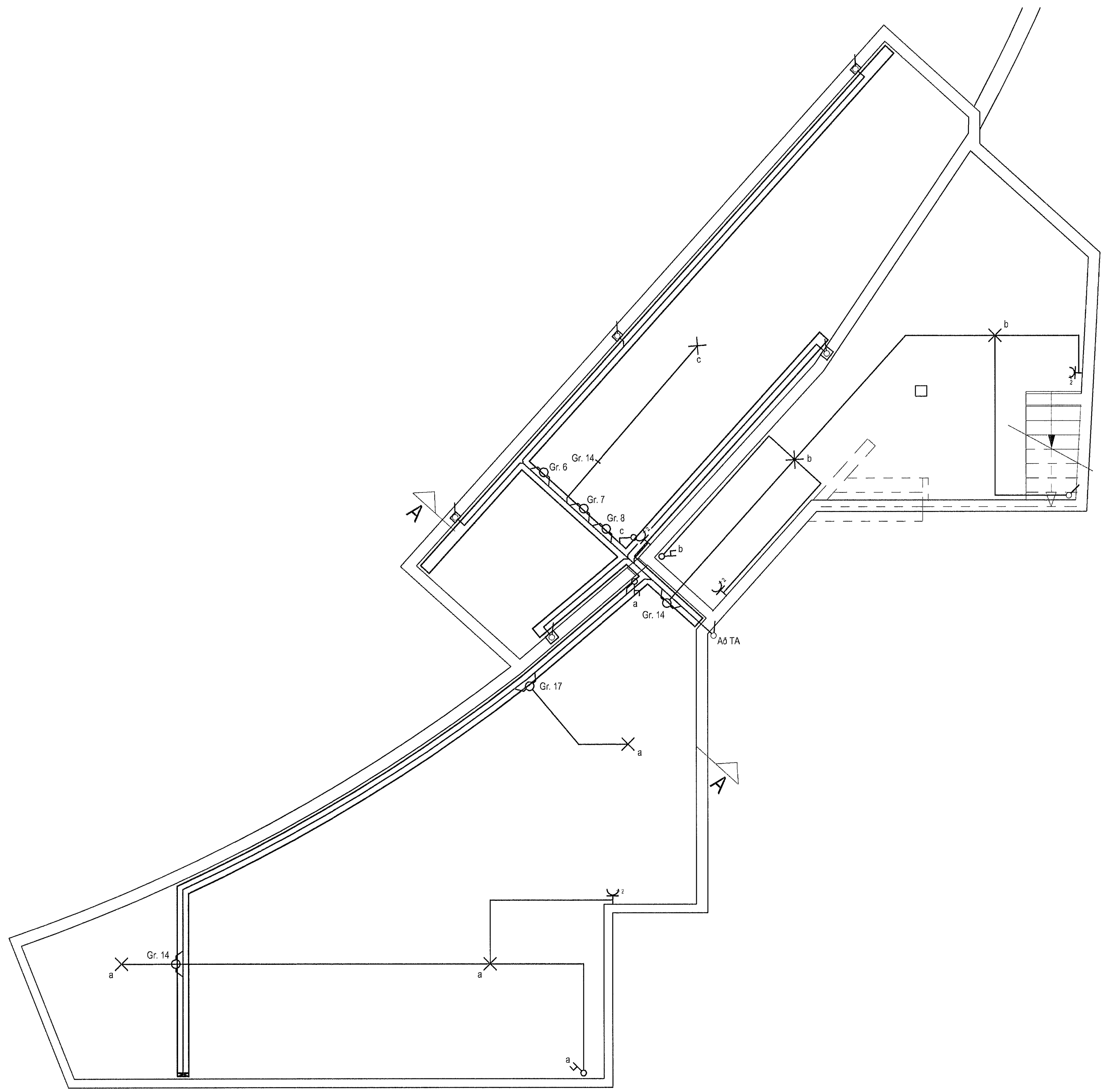
Grunnmynd, lágspennulagnir, mkv. 1:50
