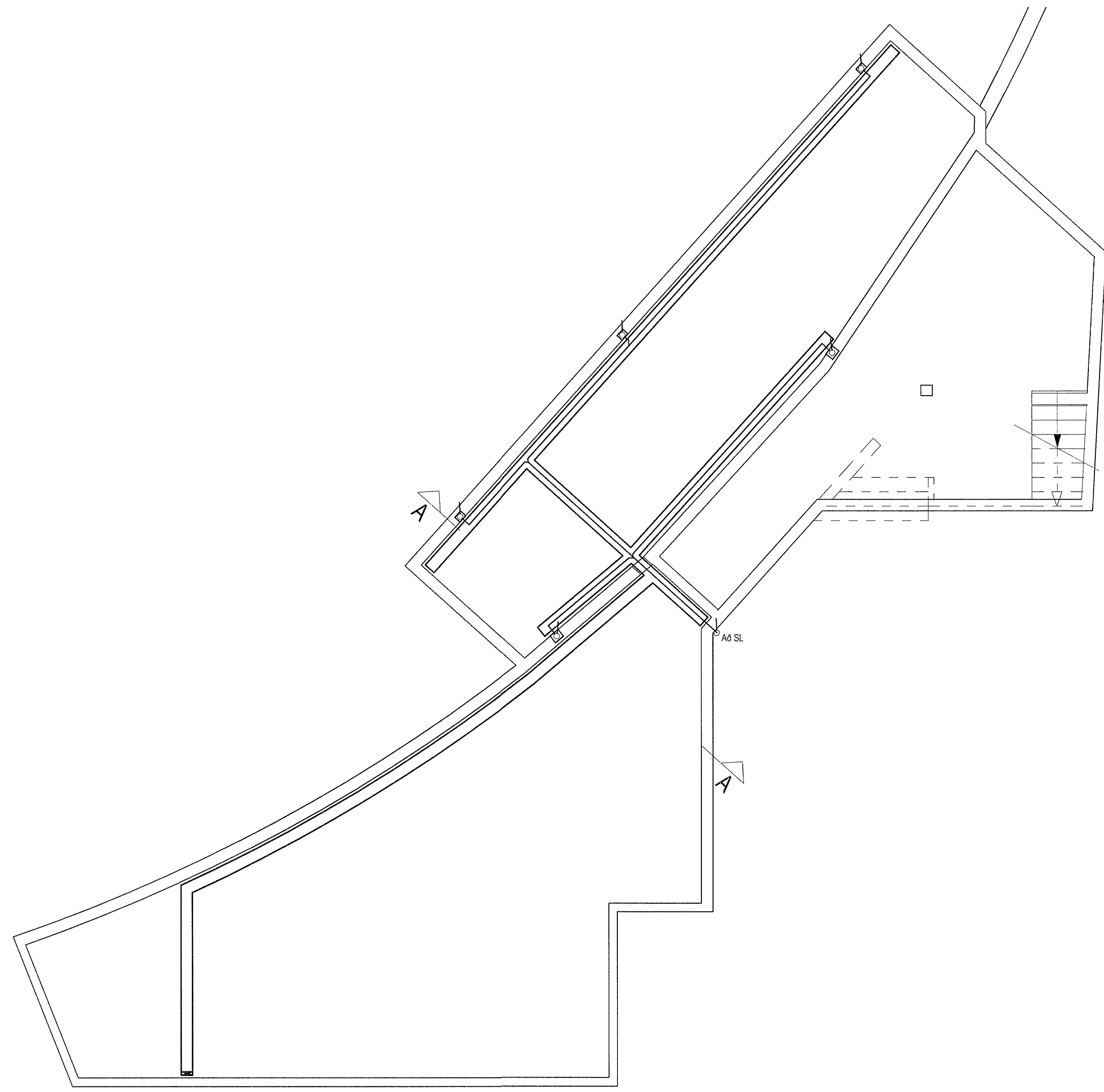
Grunnmynd, smáspennulagnir, mkv. 1:50
