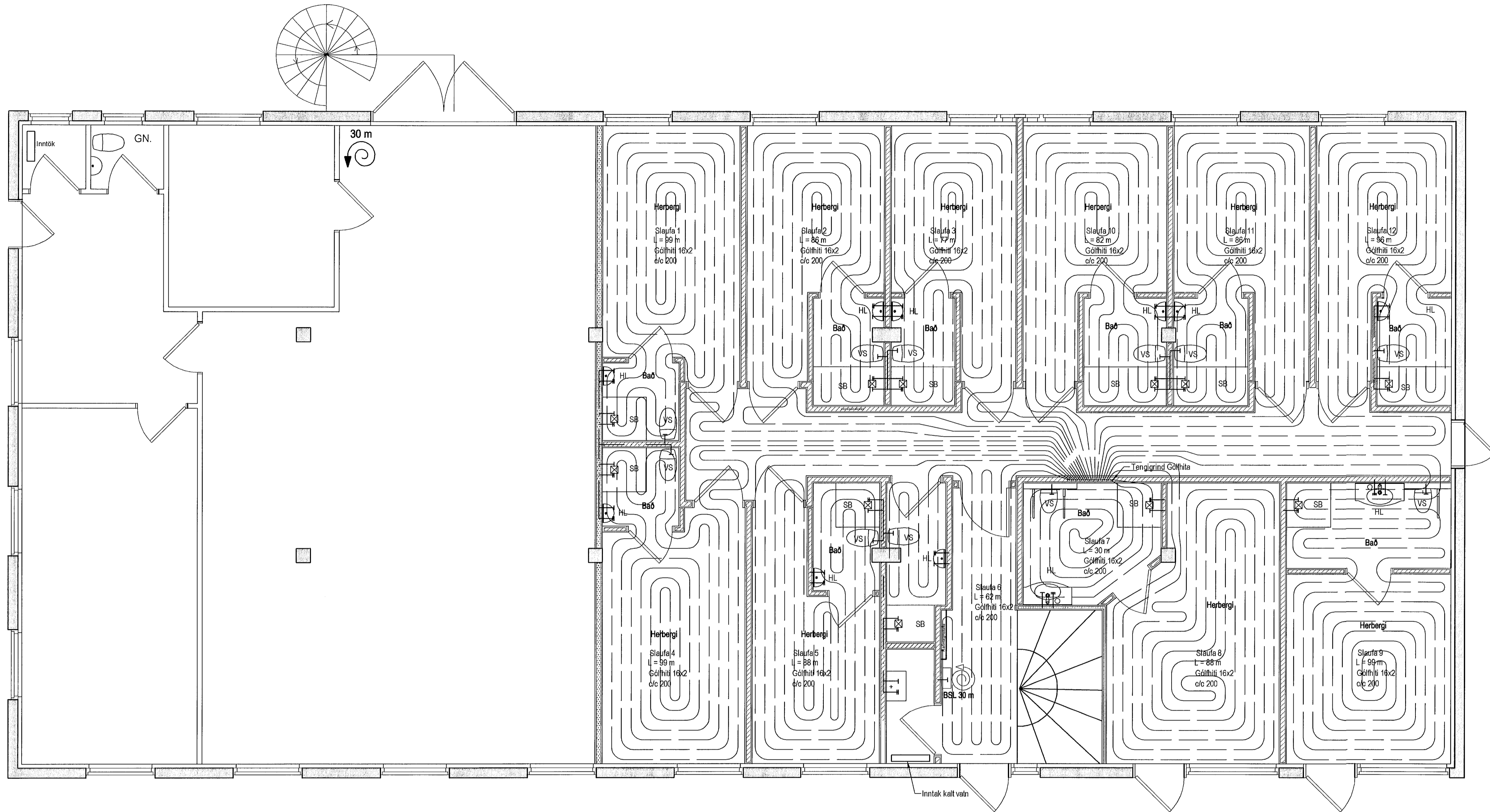
Gölfhiti 1. hæð, Grunnmynd, 1:50
