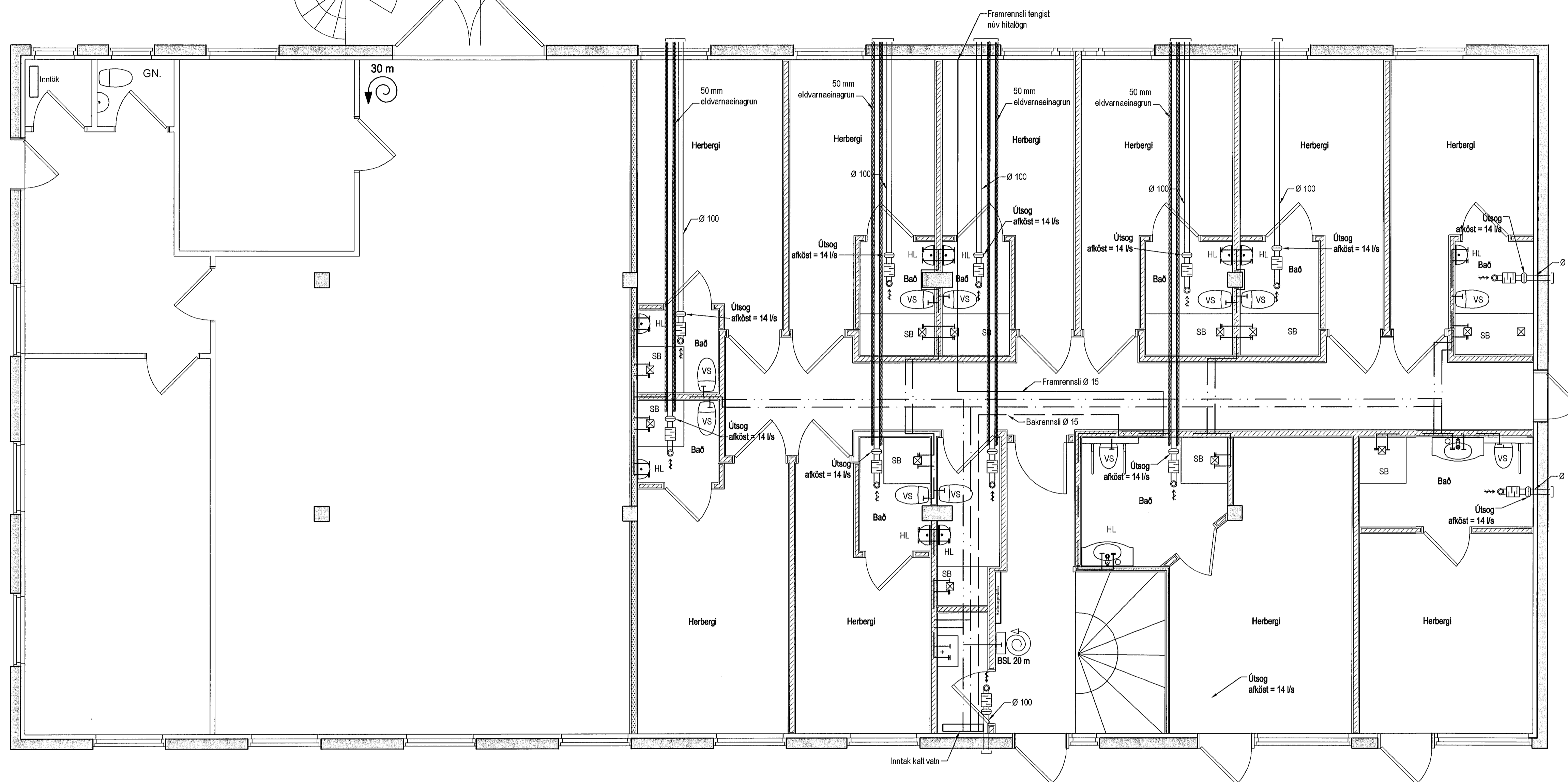
Lagnir 1. Hæð, Grunnmynd, 1:50
