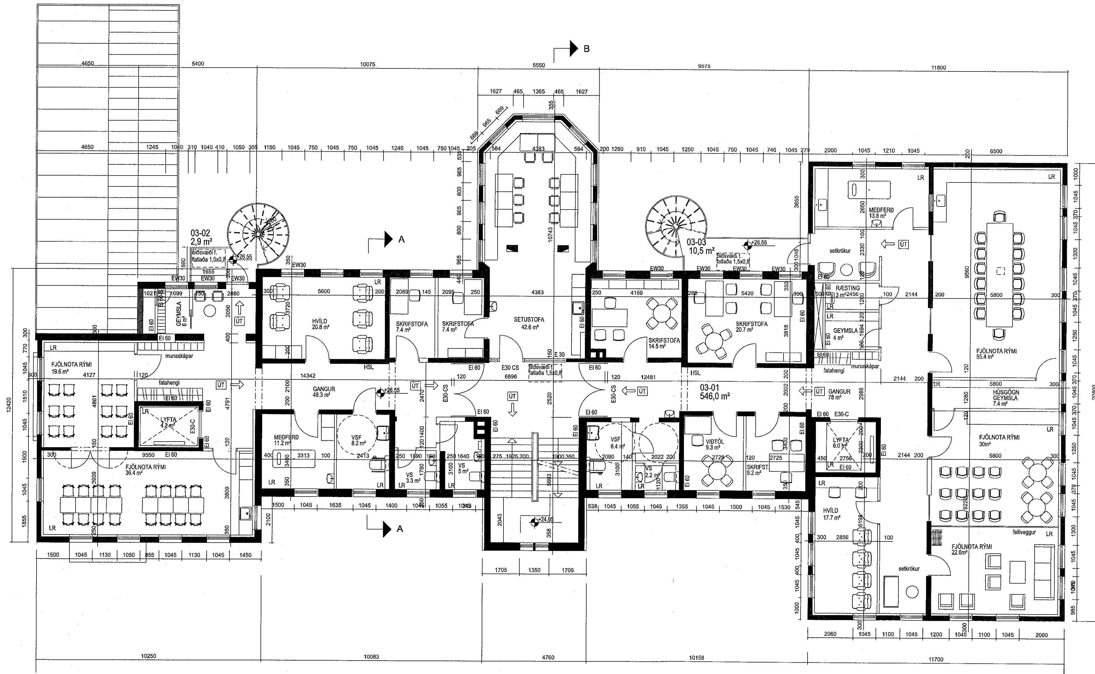
GRUNNMÝND 3. HÆÐ MKV 1:100
