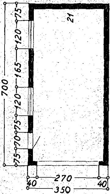
Grunnmynd
