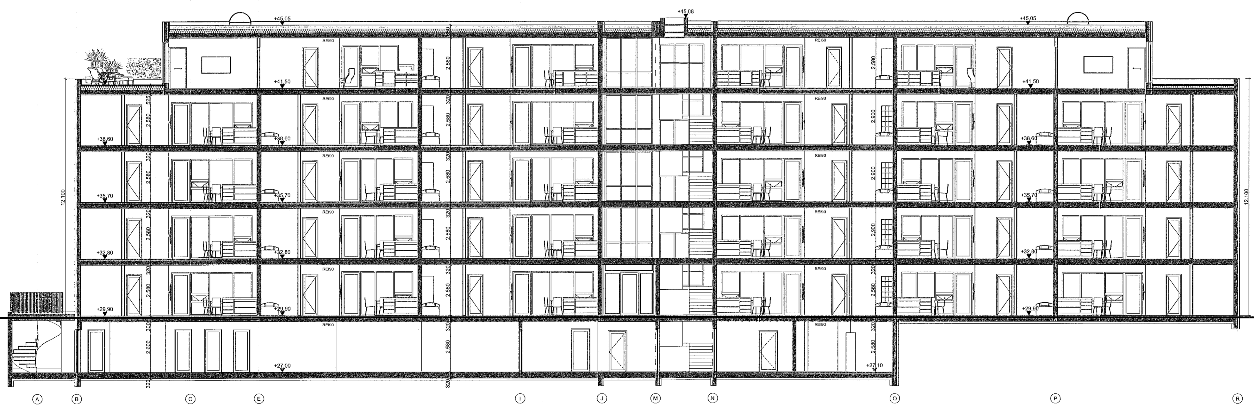
Snið C-C
