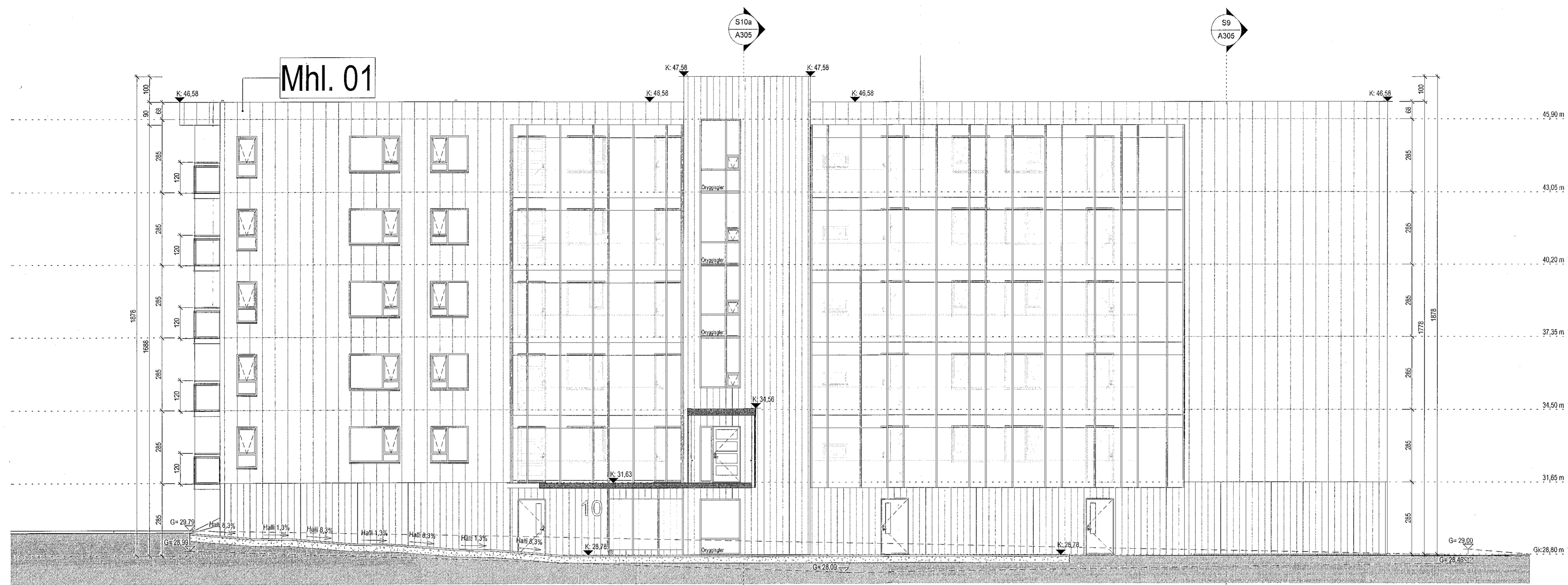
Austur útlit 1:100
