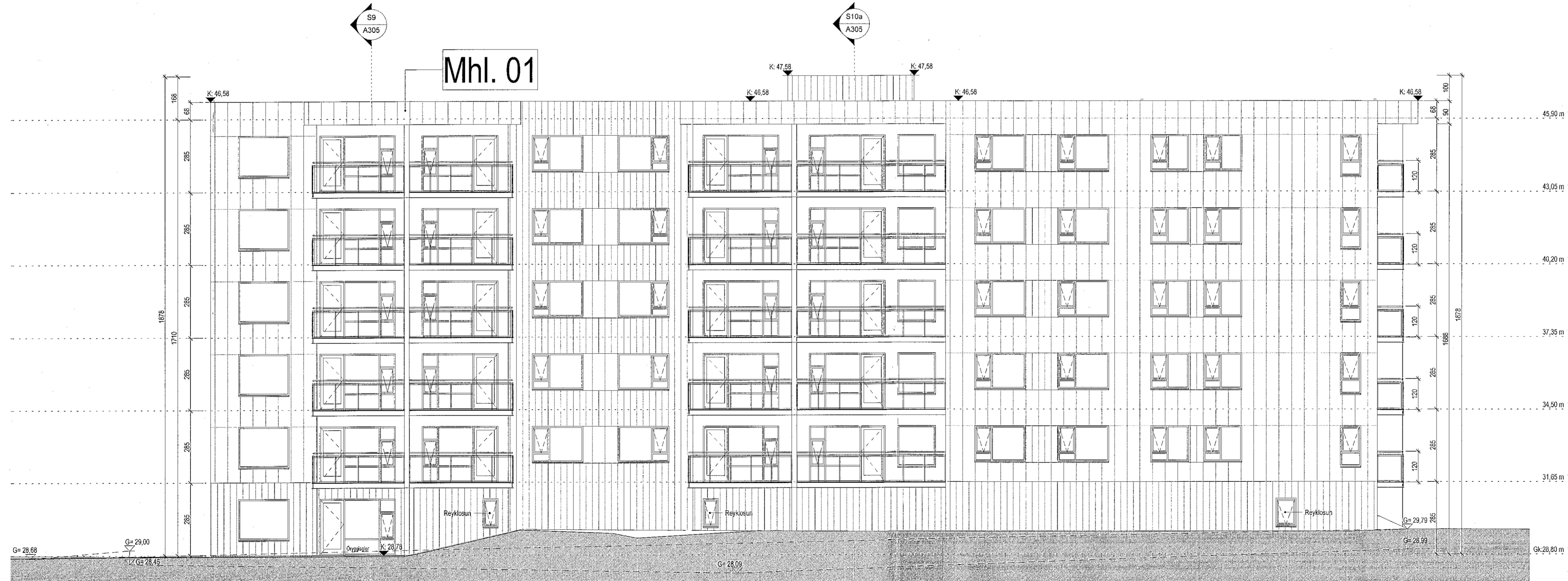
Vestur útlit 1:100
