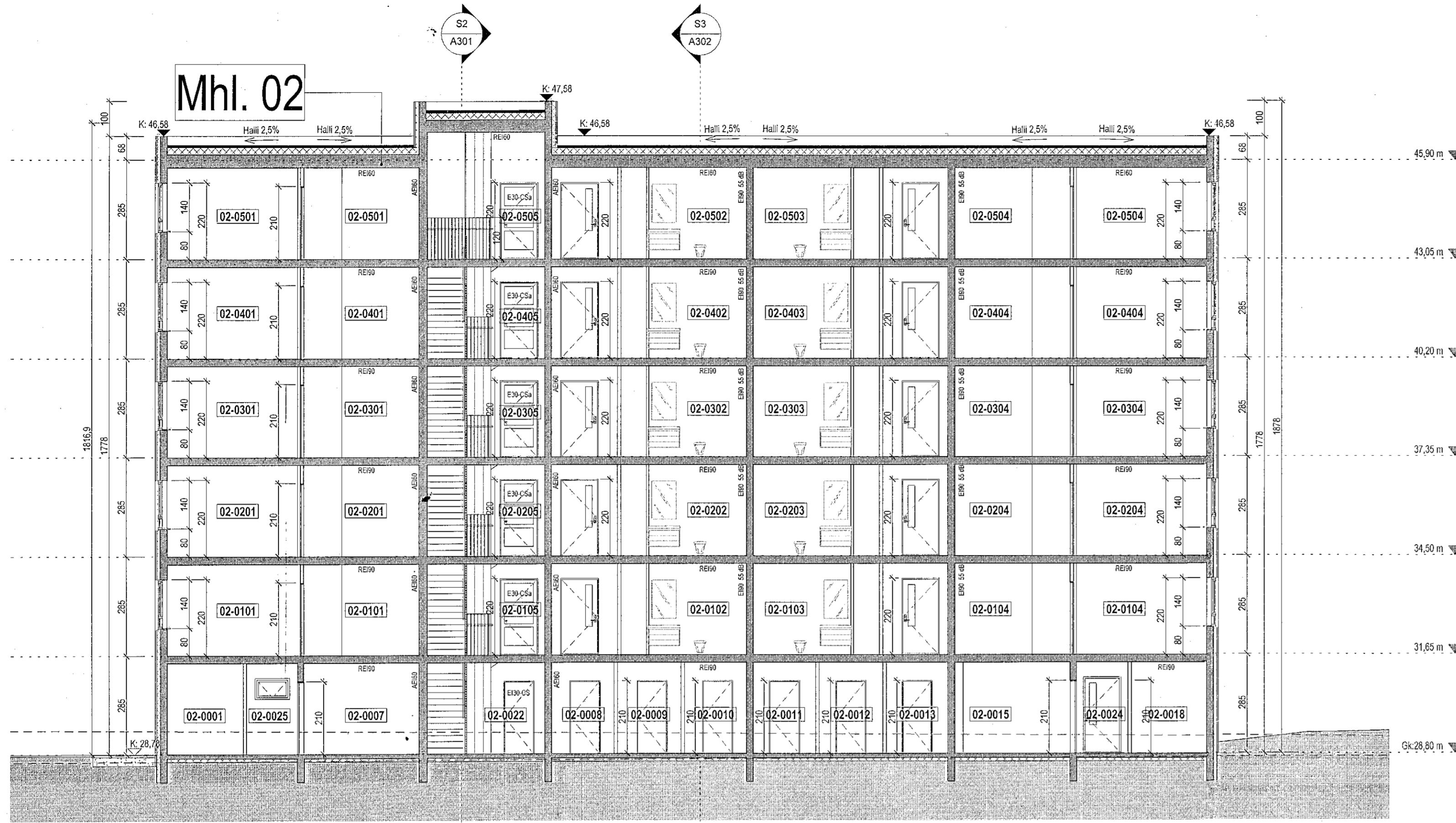
Snið 9 1:100
