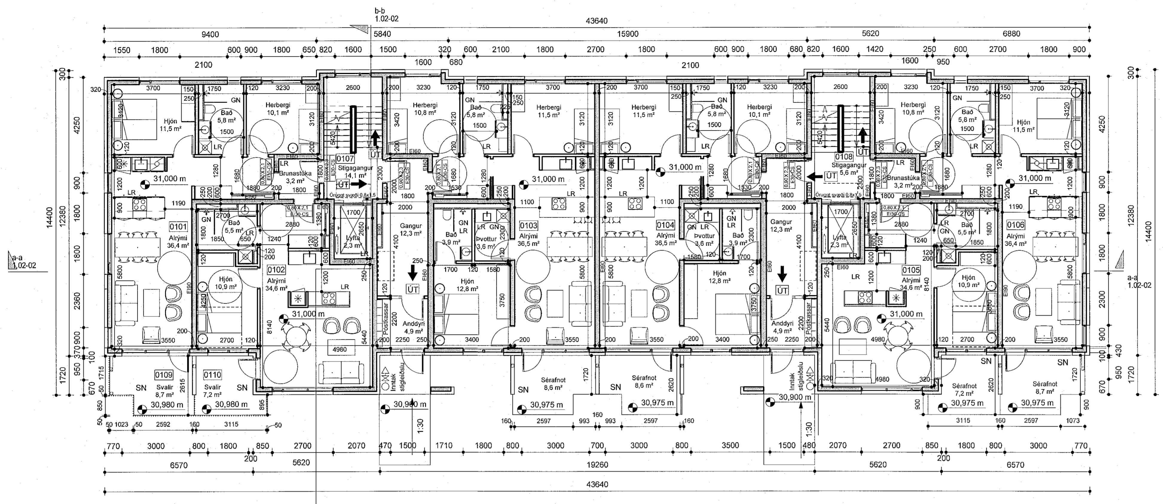
1.hæð - Áshamar 16-18 - mhl. 02 mkv: 1 : 100
