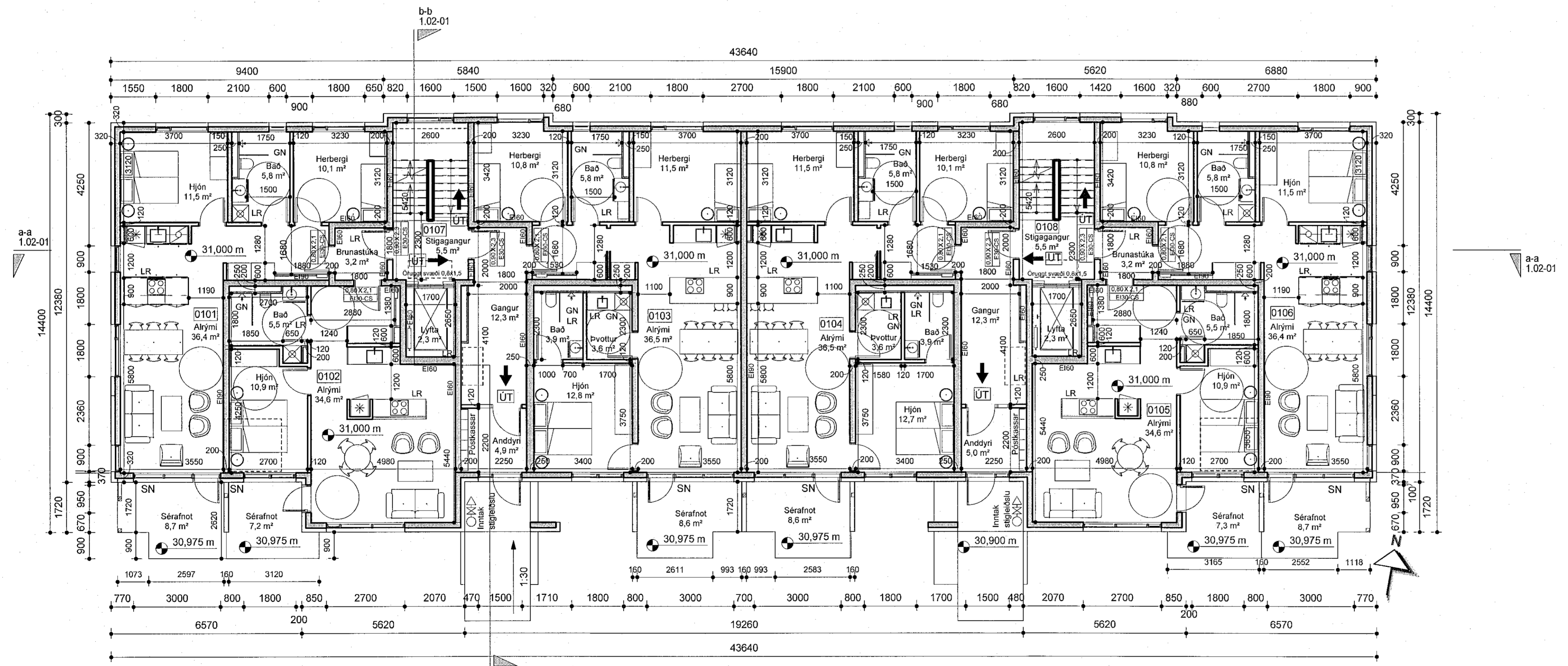
1.hæð - Áshamar 12-14 - mhl. 01 mkv: 1 : 100
