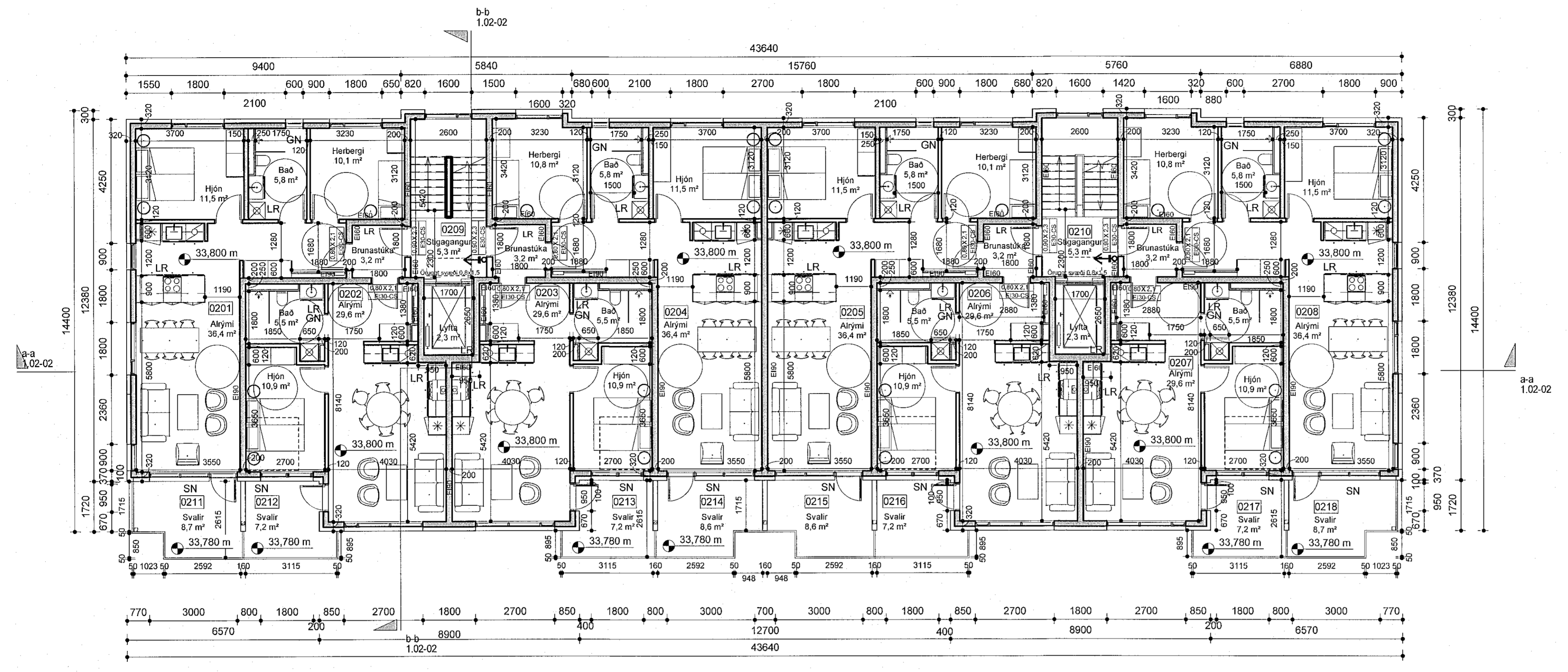
2.hæð - Áshamar 16-18 - mhl. 02 mkv: 1 : 100
