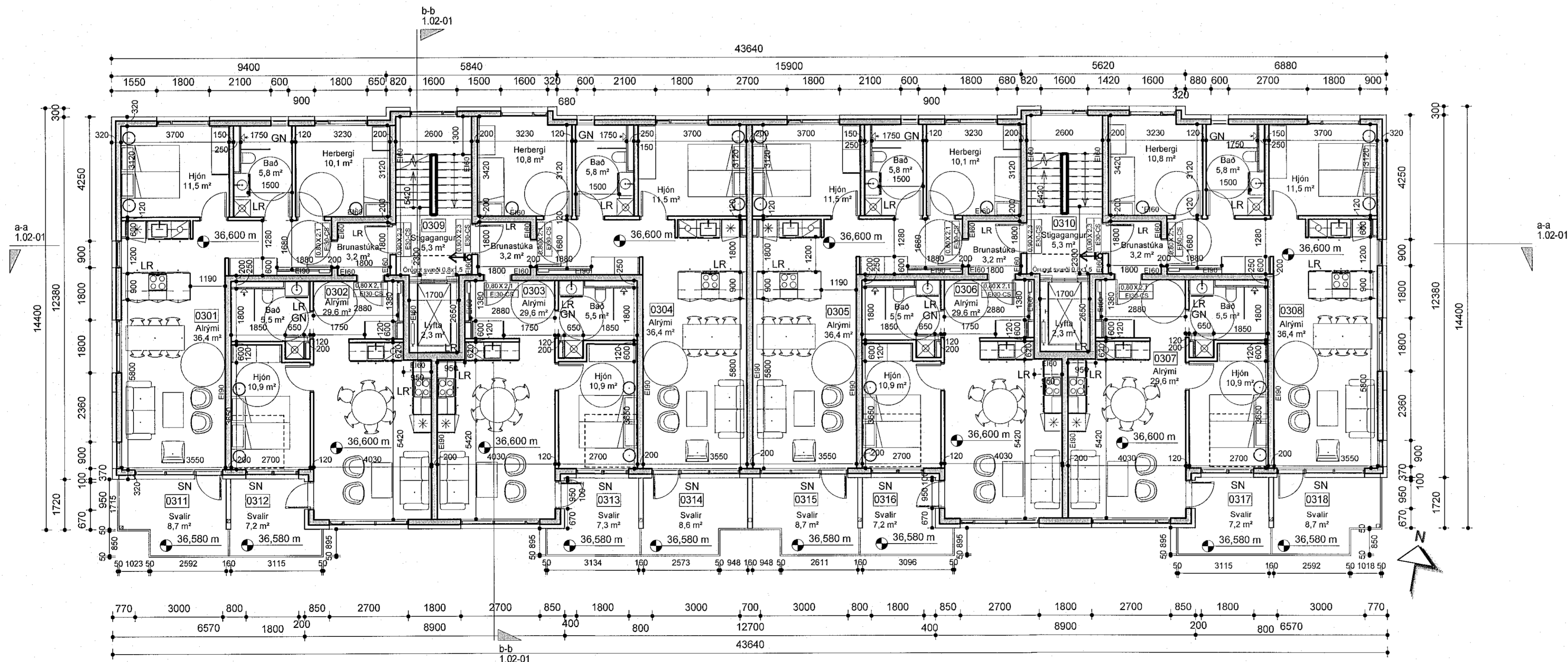
3.hæð - Áshamar 12-14 - mhl. 01 mkv: 1 : 100
