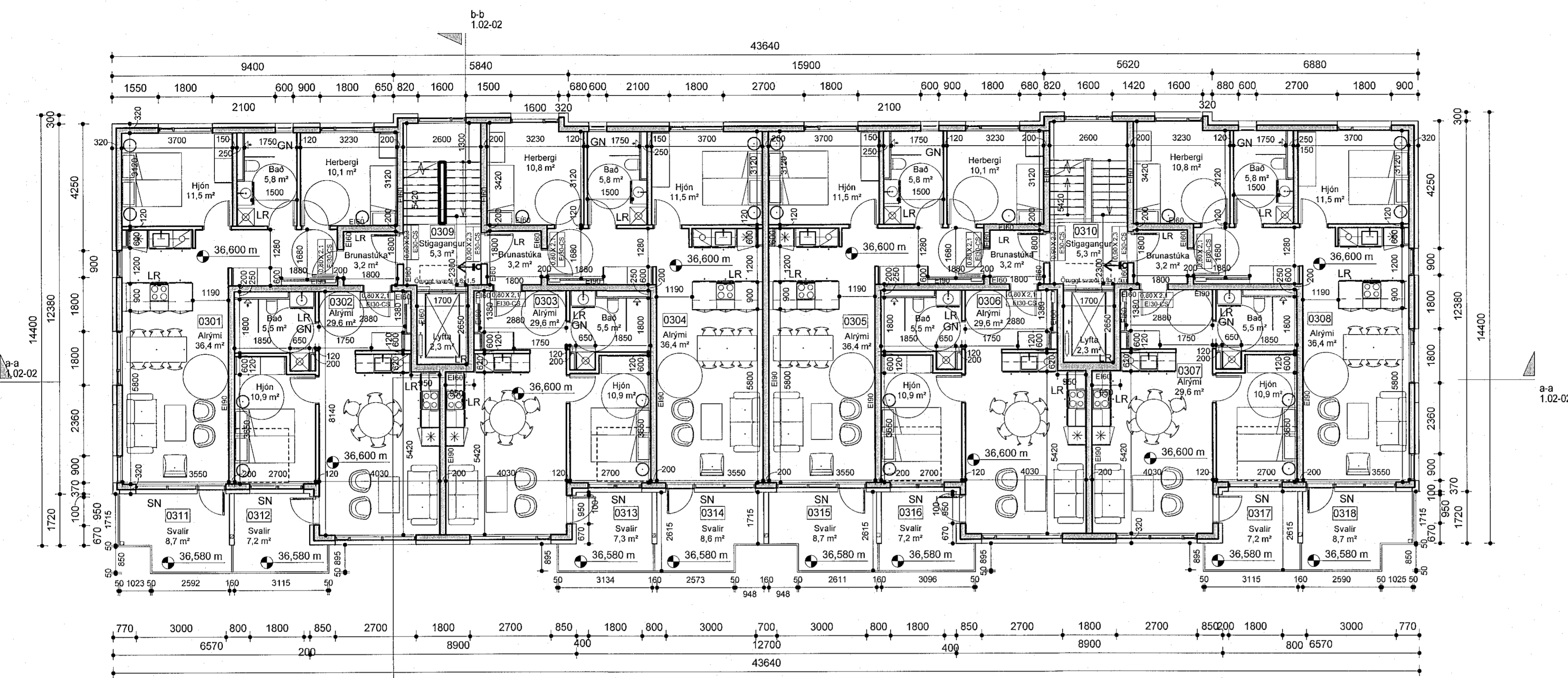
3.hæð - Áshamar 16-18 - mhl. 02 mkv: 1 : 100
