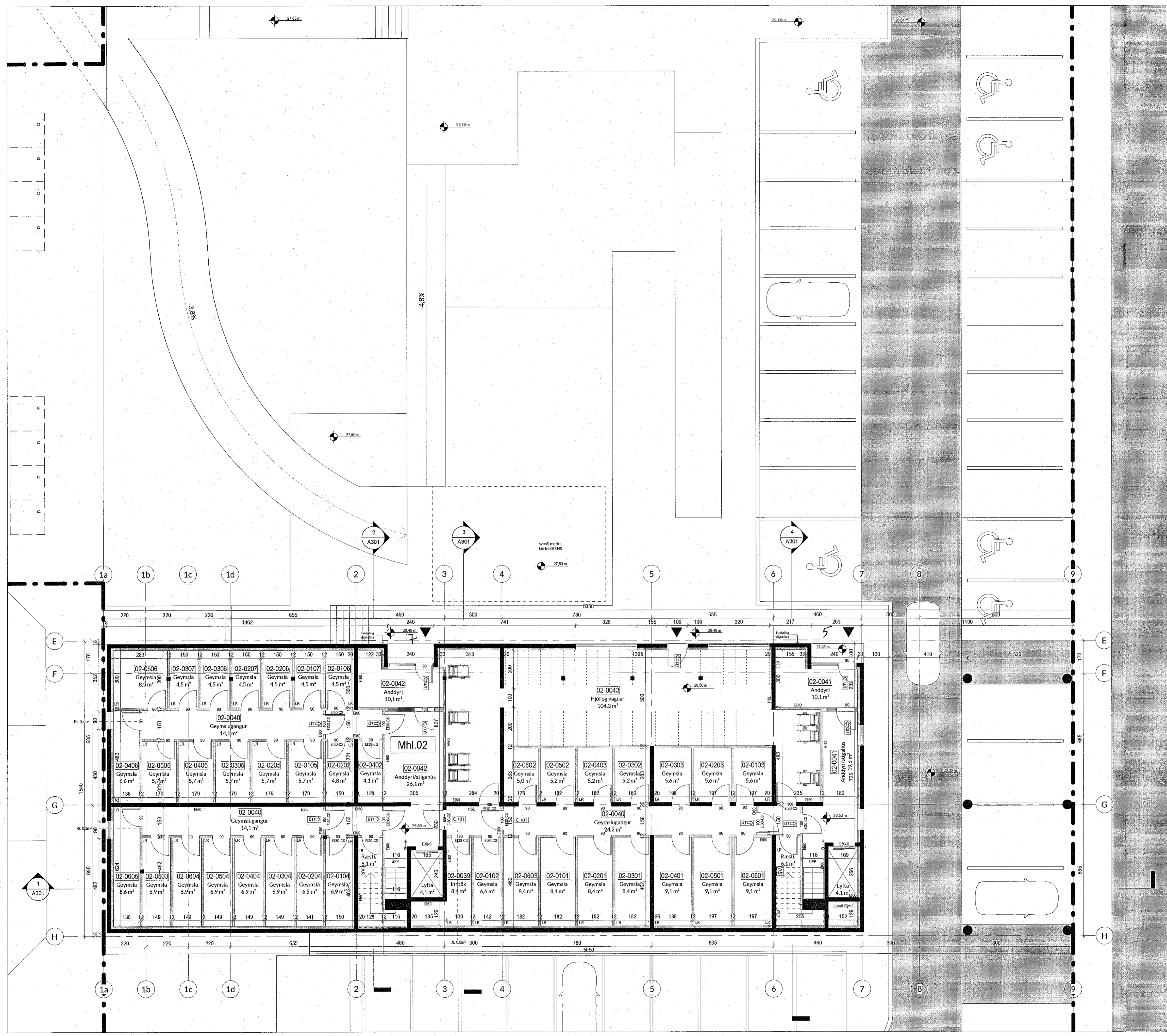
Mhl.02 Kjallari 1:100
