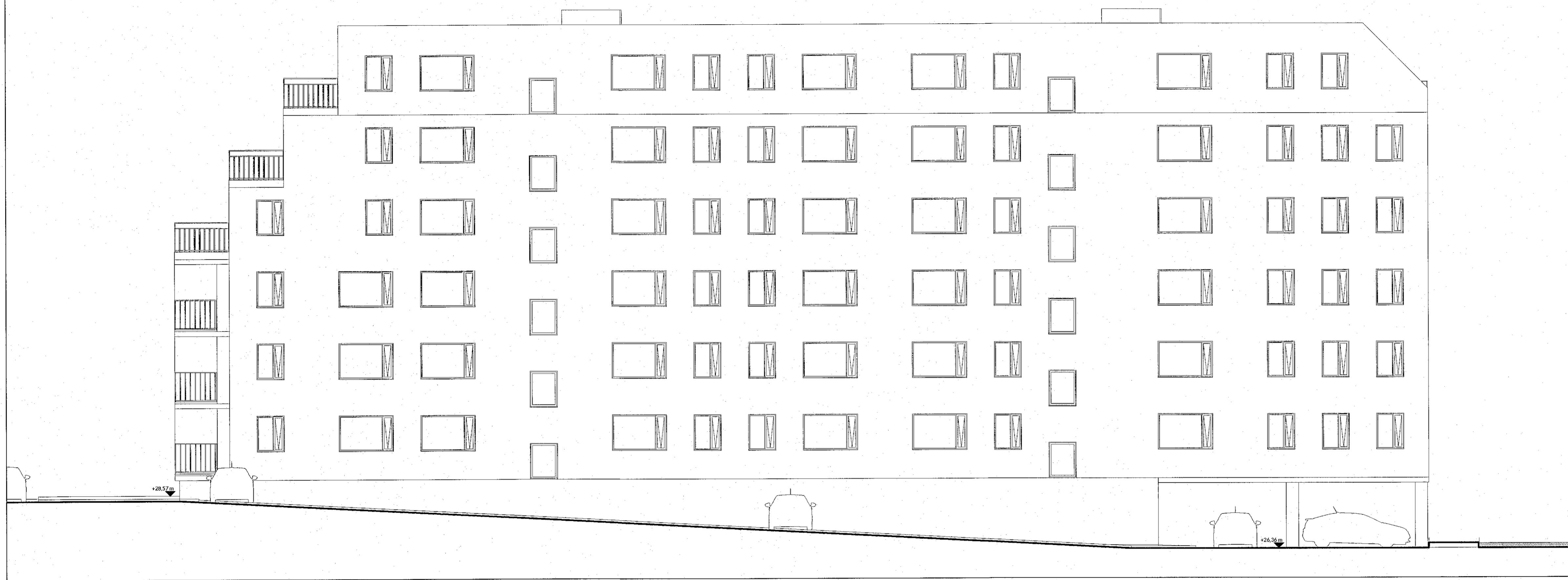
Útlit Austur Mhl.02 1:100
