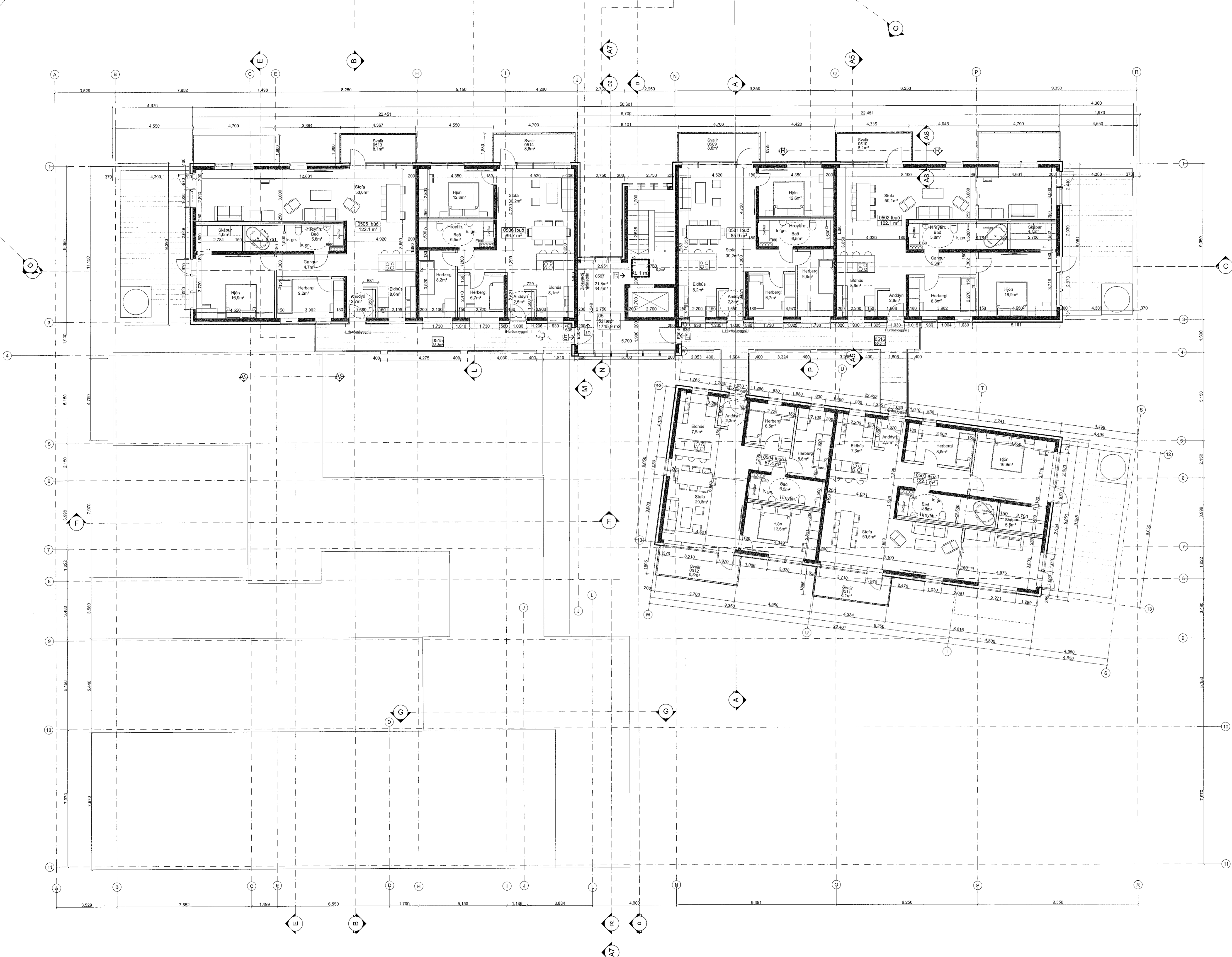
Grunnmynd 5.hæð
