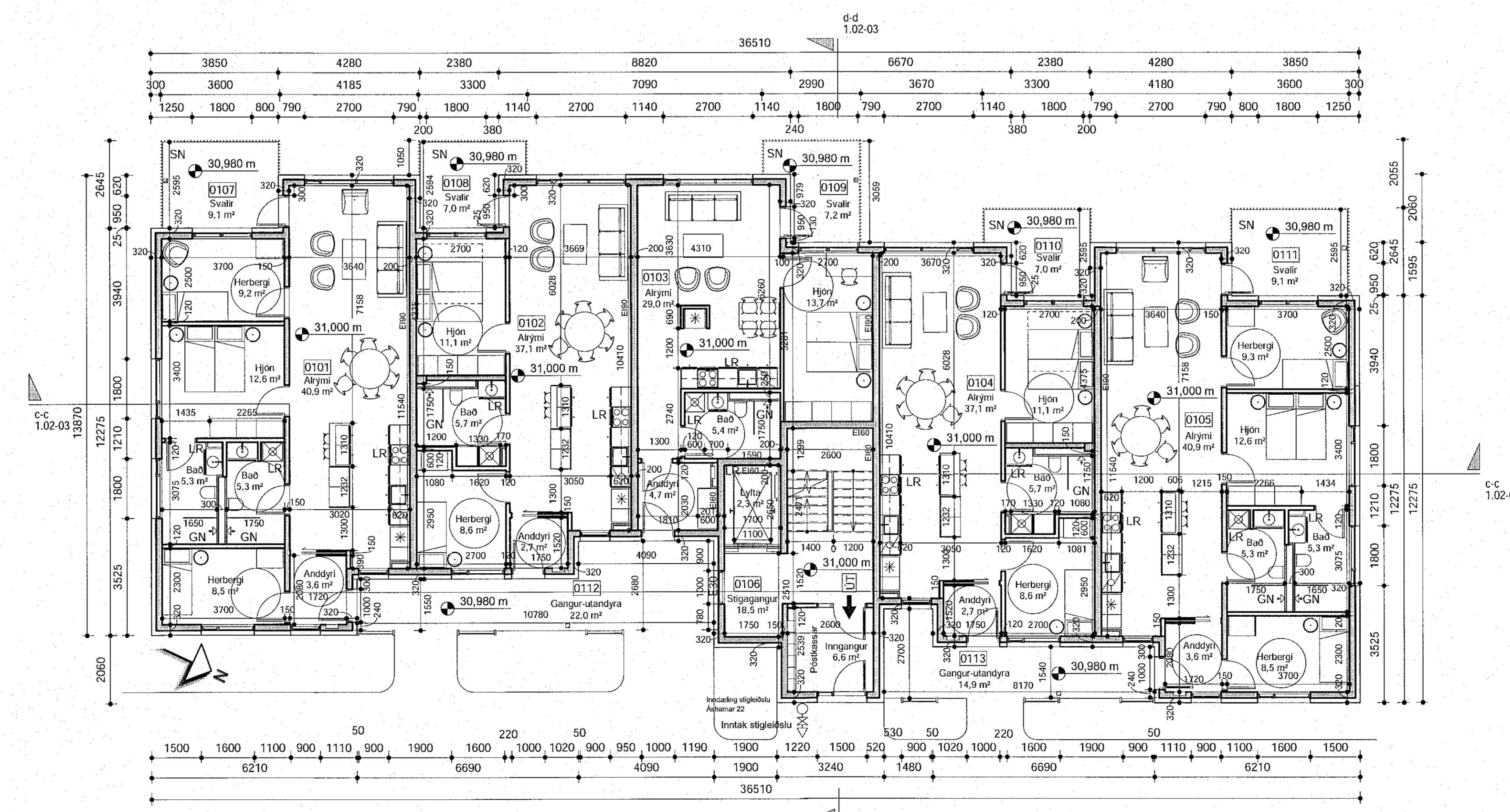
1.hæð - Áshamar 20 - mhl. 03 mkv: 1 : 100
