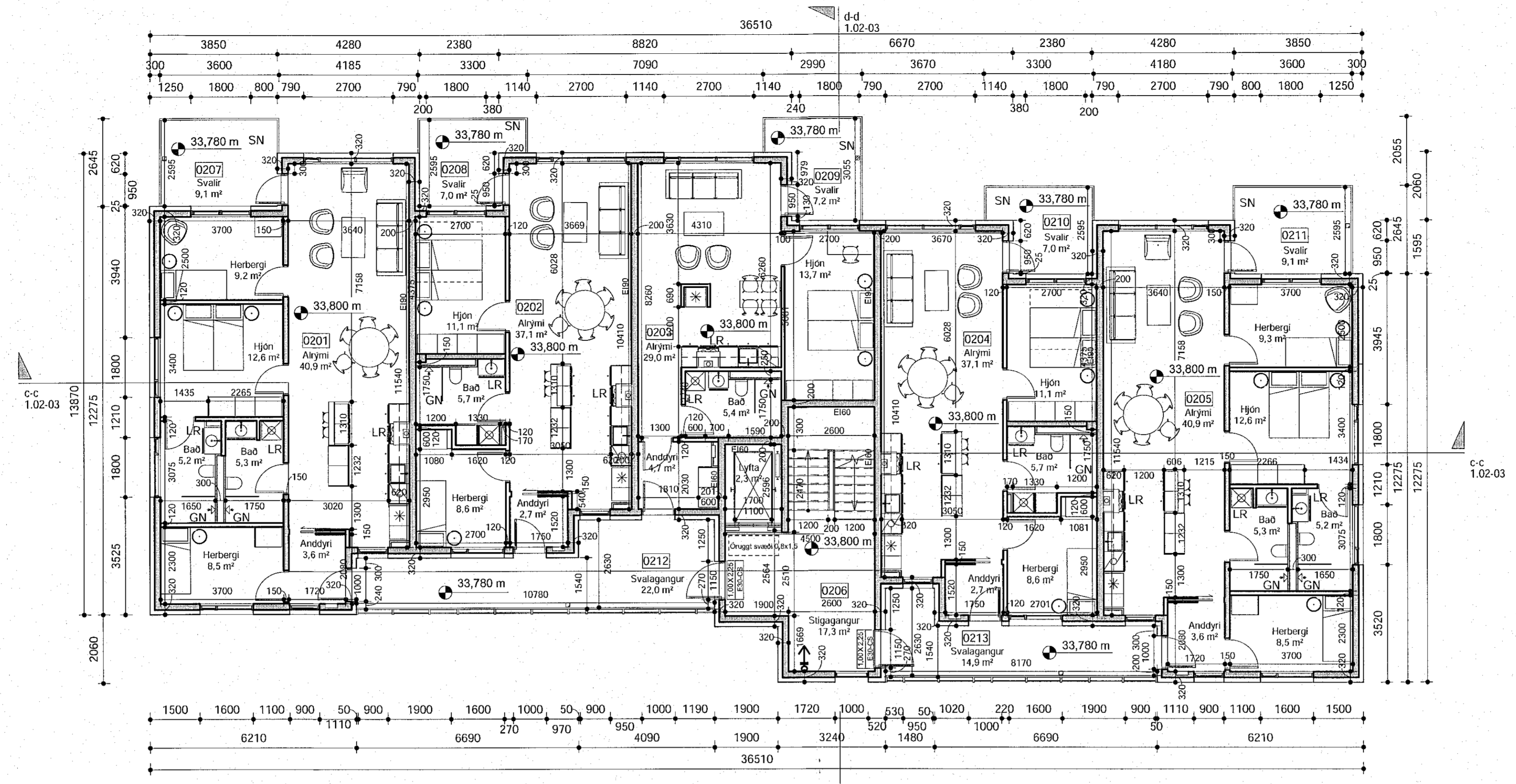
2.hæð - Áshamar 20 - mhl. 03 mkv: 1 : 100
