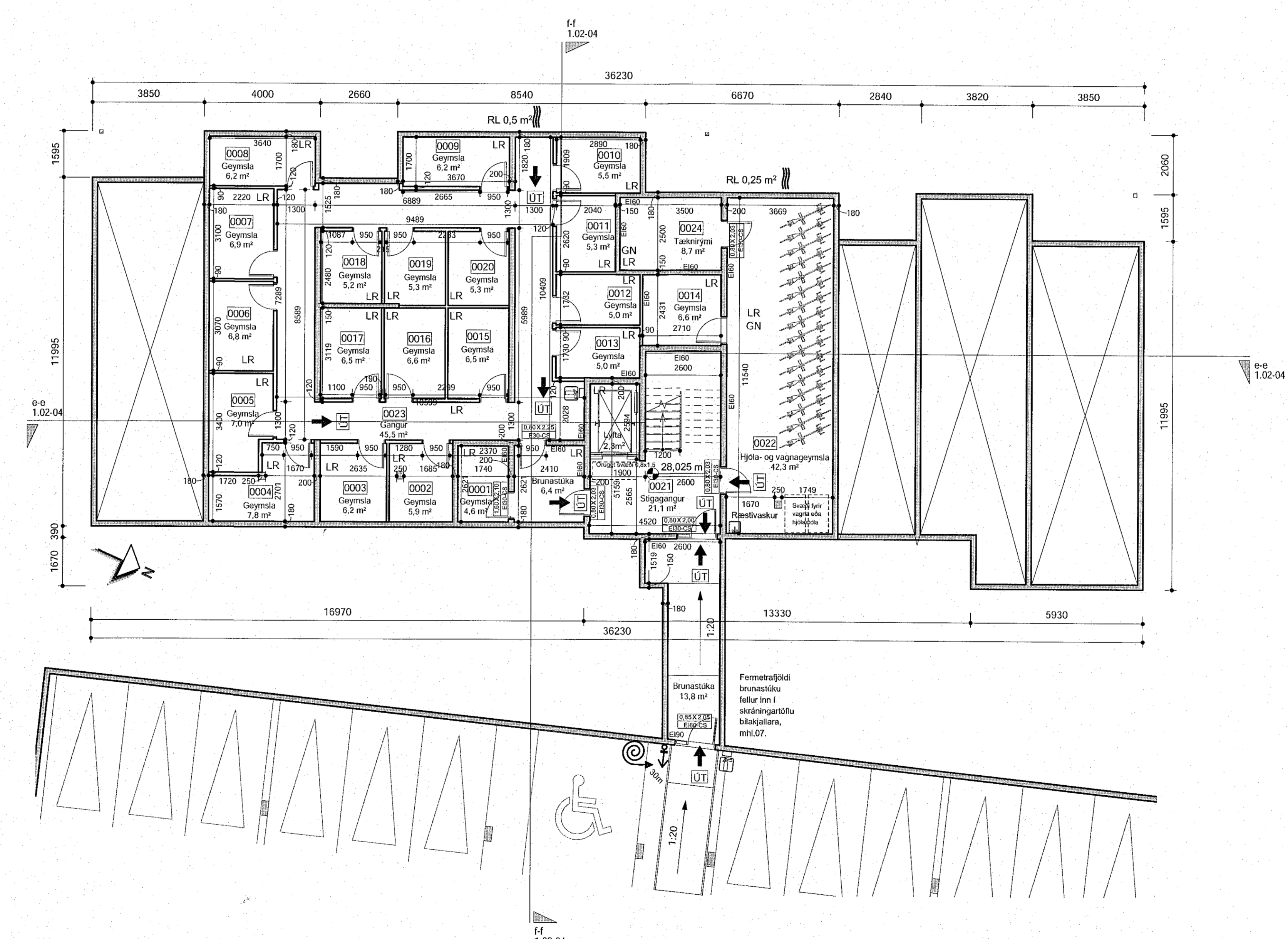
0.Kjallari - Áshamar 22 - mhl.04 mkv: 1 : 100
