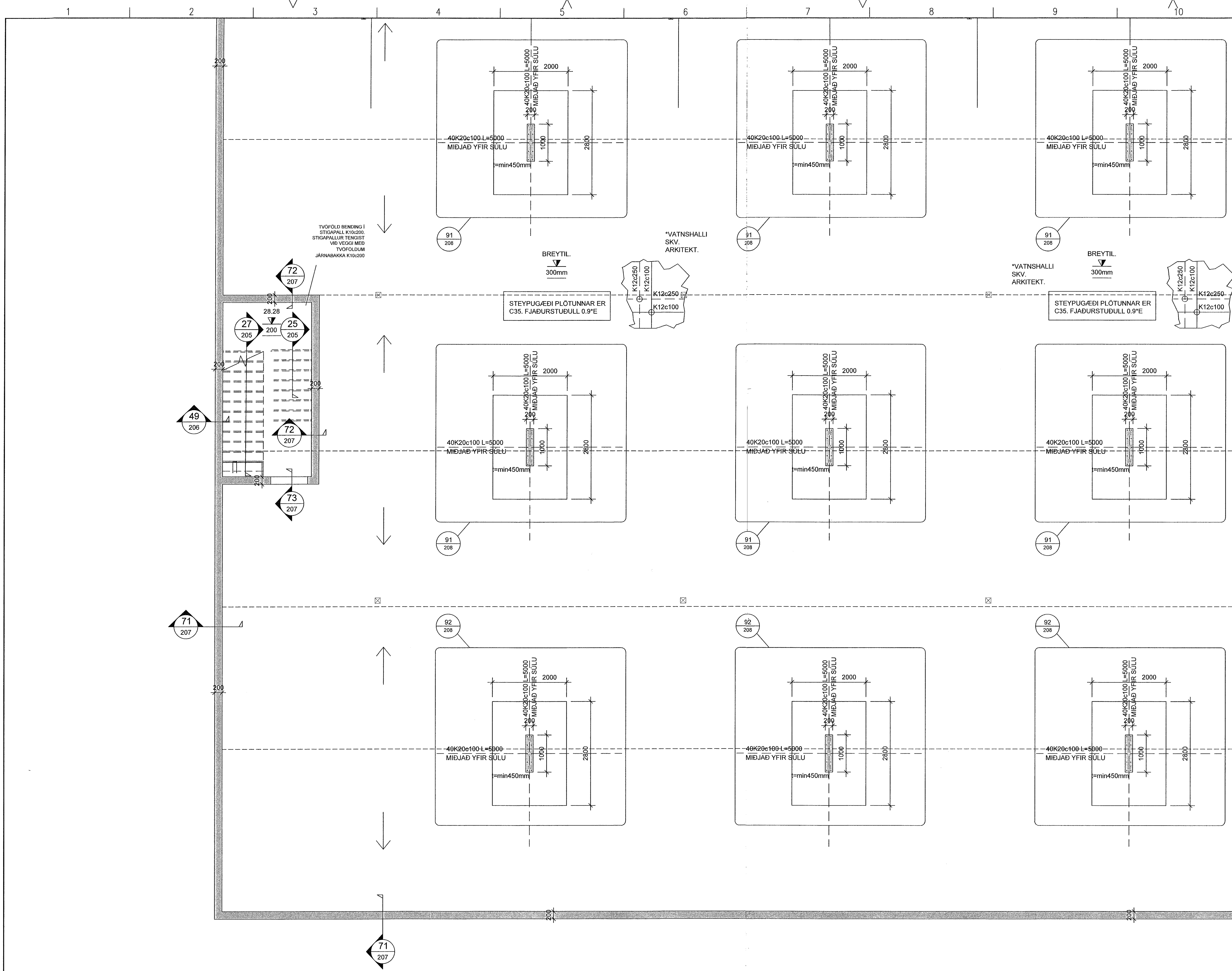
VEGGIR OG LOFTAPLATA KJALLARA, GRUNNMYND MKV. 3
