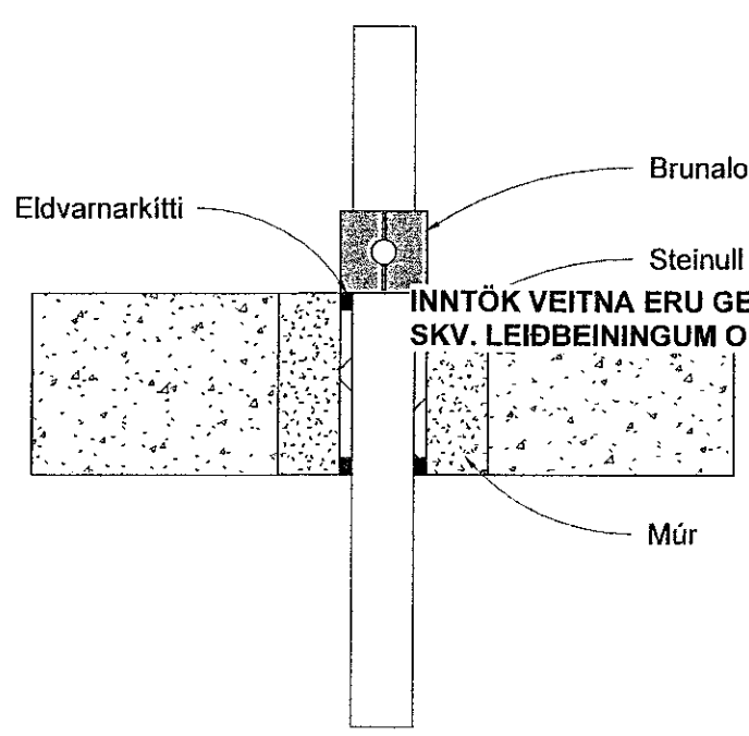
Brunapétting á loftræstilögn í gegnum steipt gólf utan lagnaskakts
