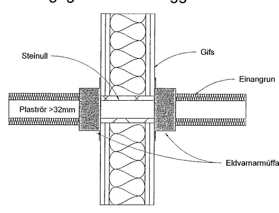
Brunapétting á plastlögn stærri en Ø32mm í gegnum léttan vegg
