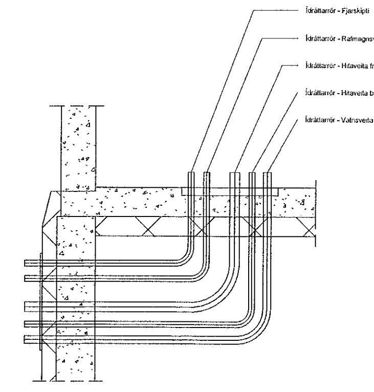
FRÁGANGUR INNTÖK VEITNA
