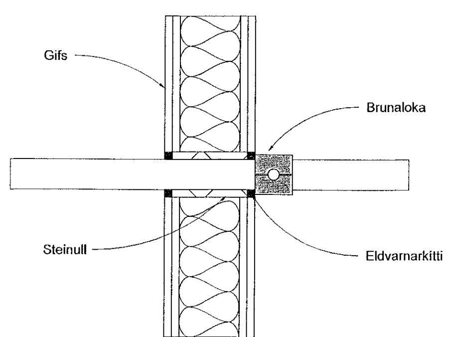
Brunapétting á loftræstilögn í gegnum léttan vegg
