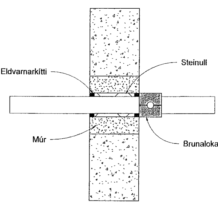
Brunapétting á loftræstilögn í gegnum steiptan vegg
