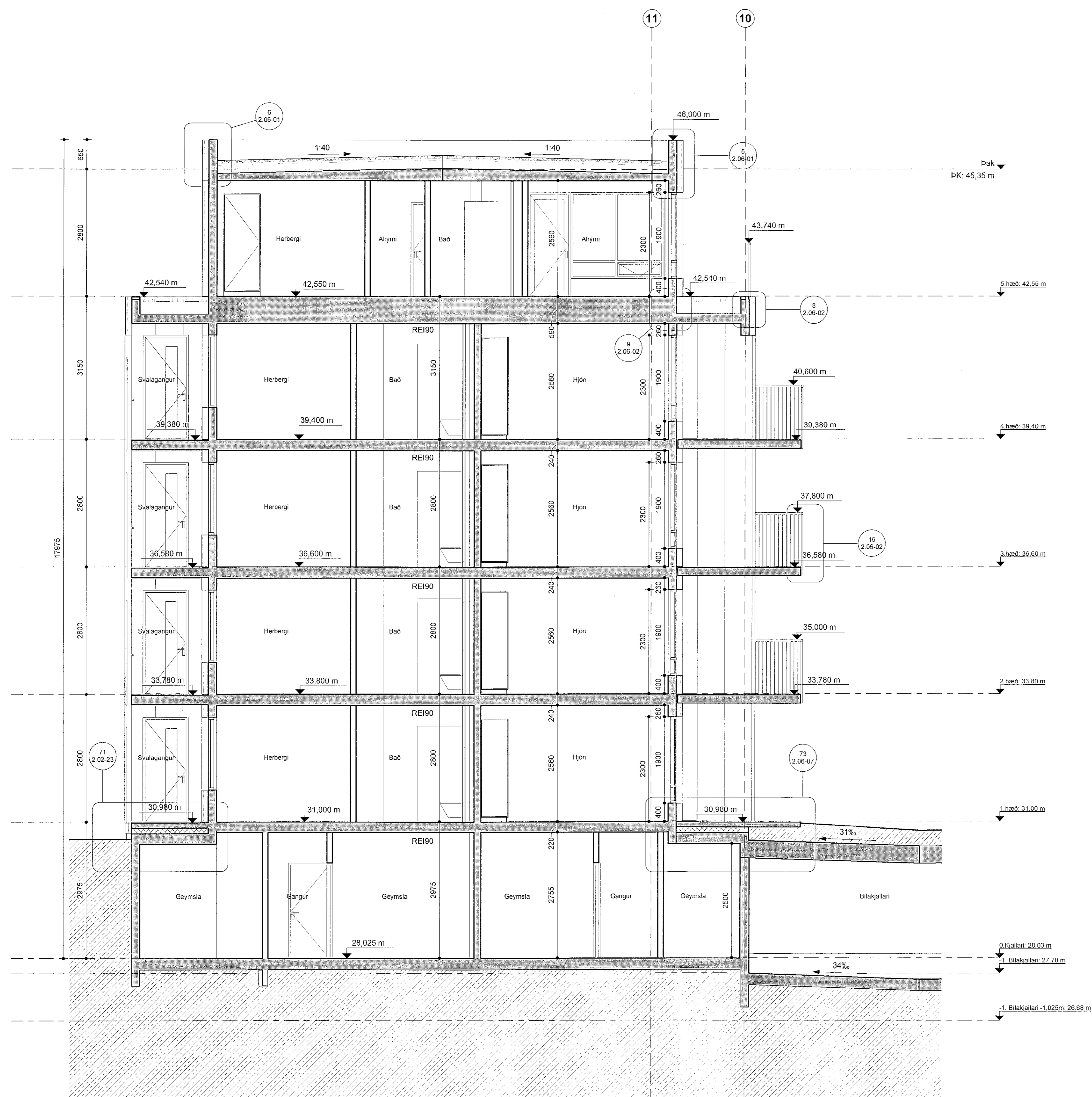
Áshamar 26 mhl.06 - snið o-o mkv: 1 : 50
